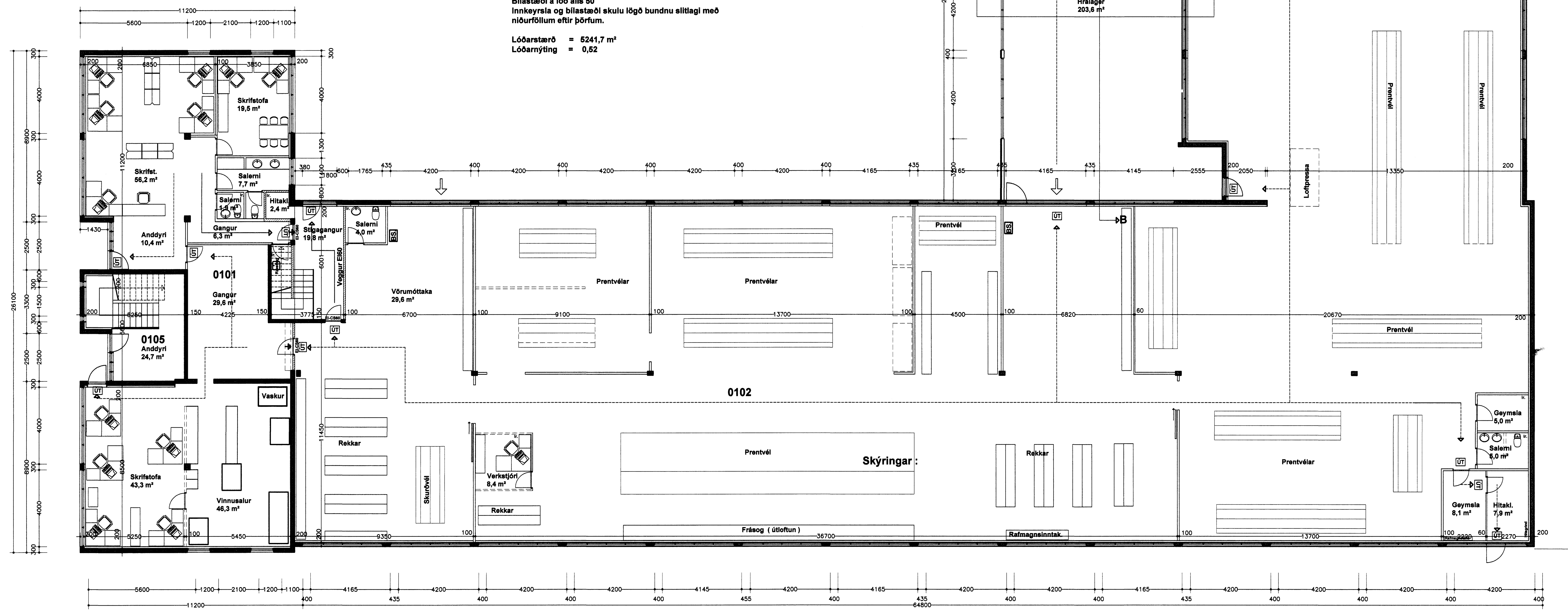
Grunnmynd 1. hæðar.
