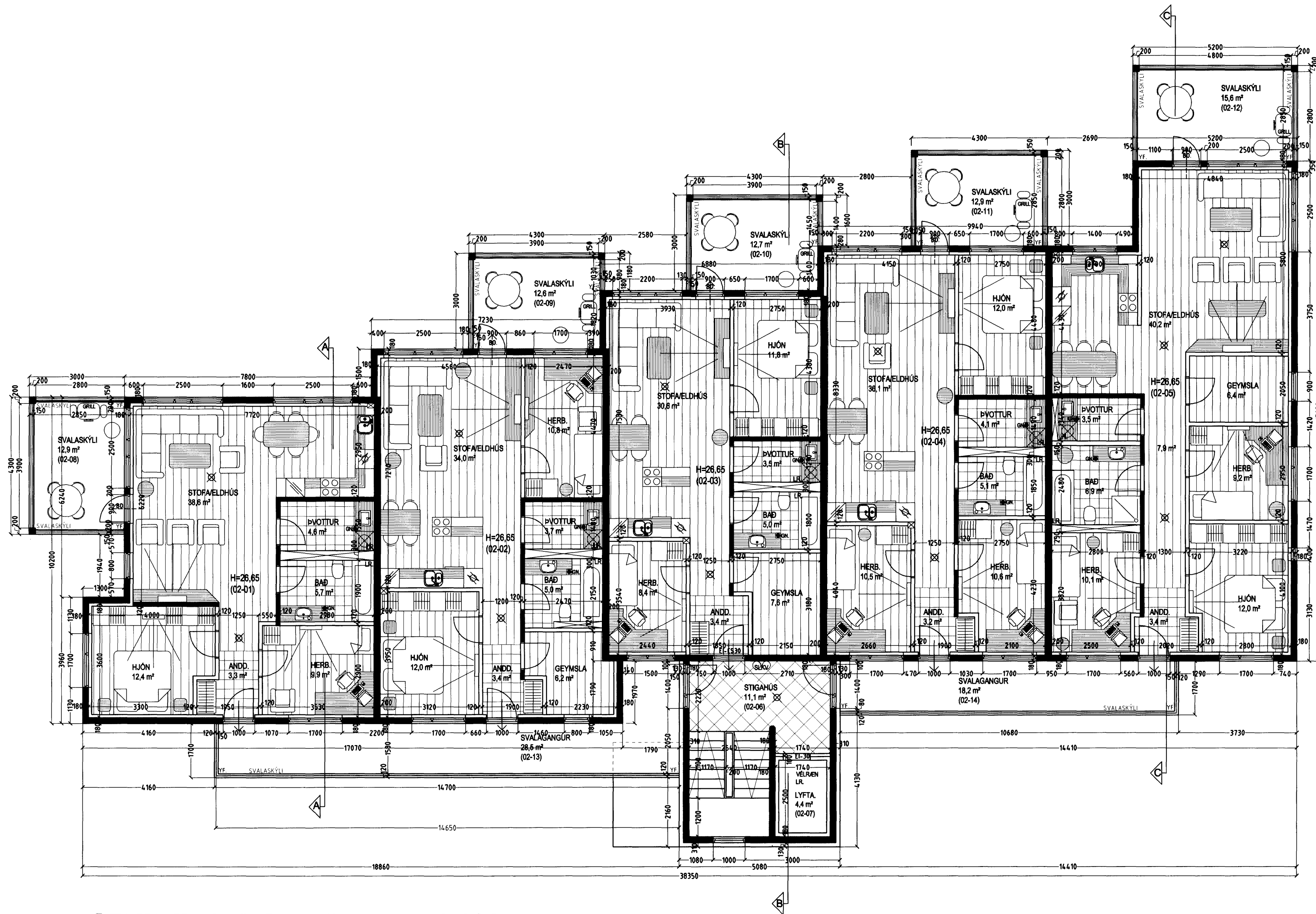
GRUNNMYND 2. HÆÐ MKV. 1:100.
