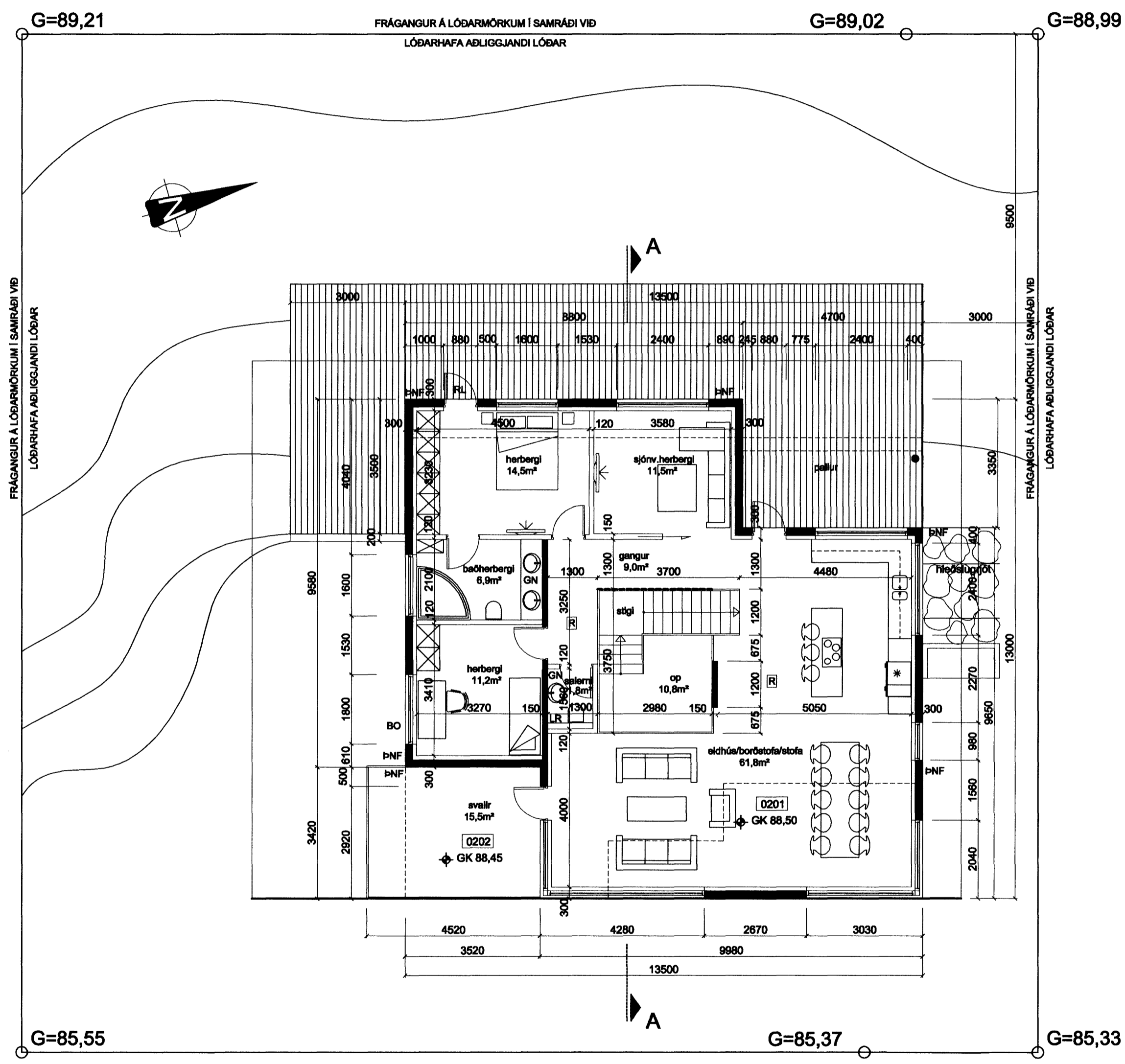
GRUNNMYND 2. HÆÐ 1:100
