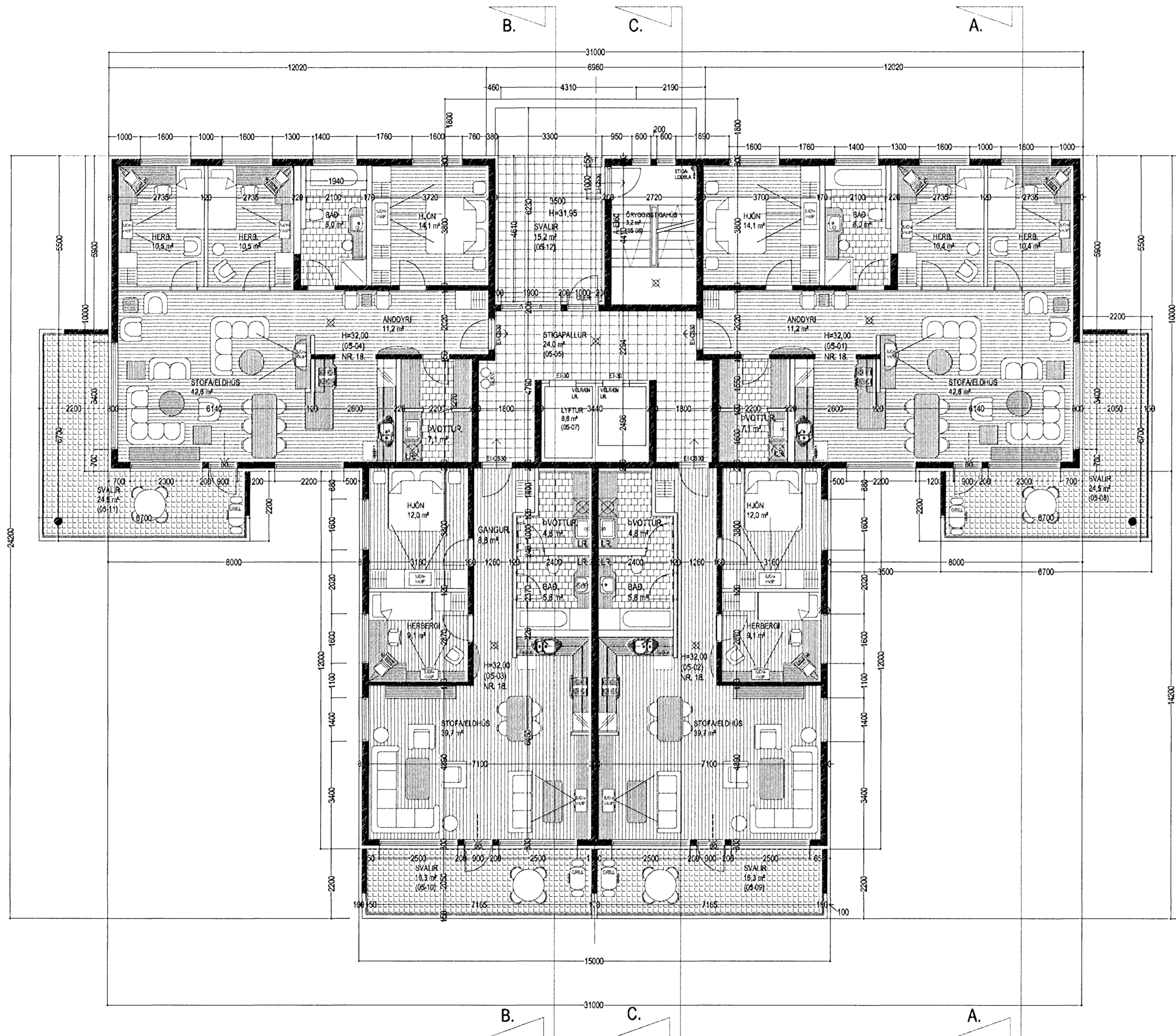
GRUNNMYND 5. HÆÐ MKV. 1:100.
