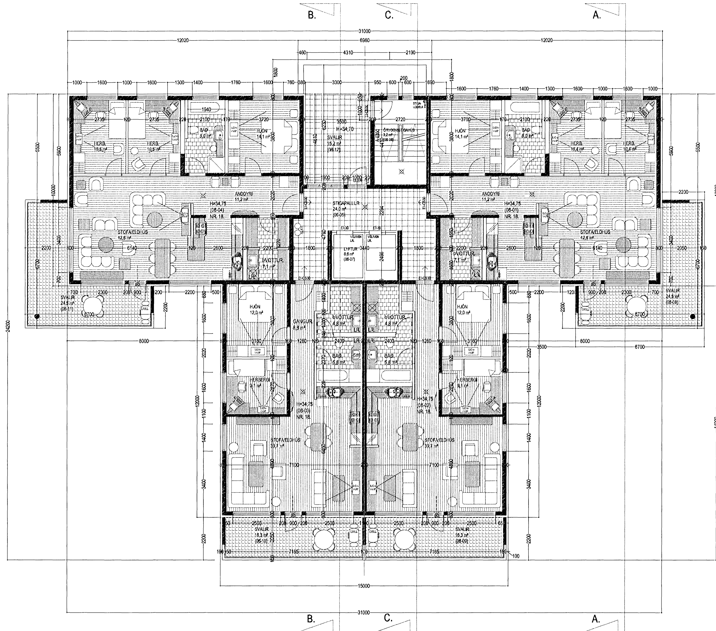
GRUNNMYND 6. HÆÐ MKV. 1:100.
