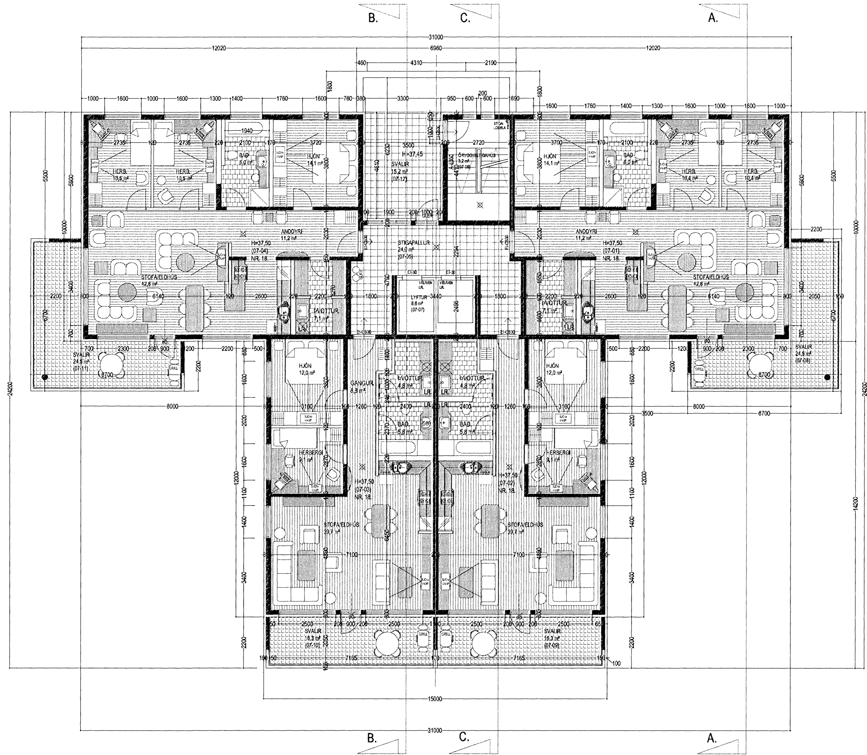
GRUNNMYND 7. HÆÐ MKV. 1:100.
