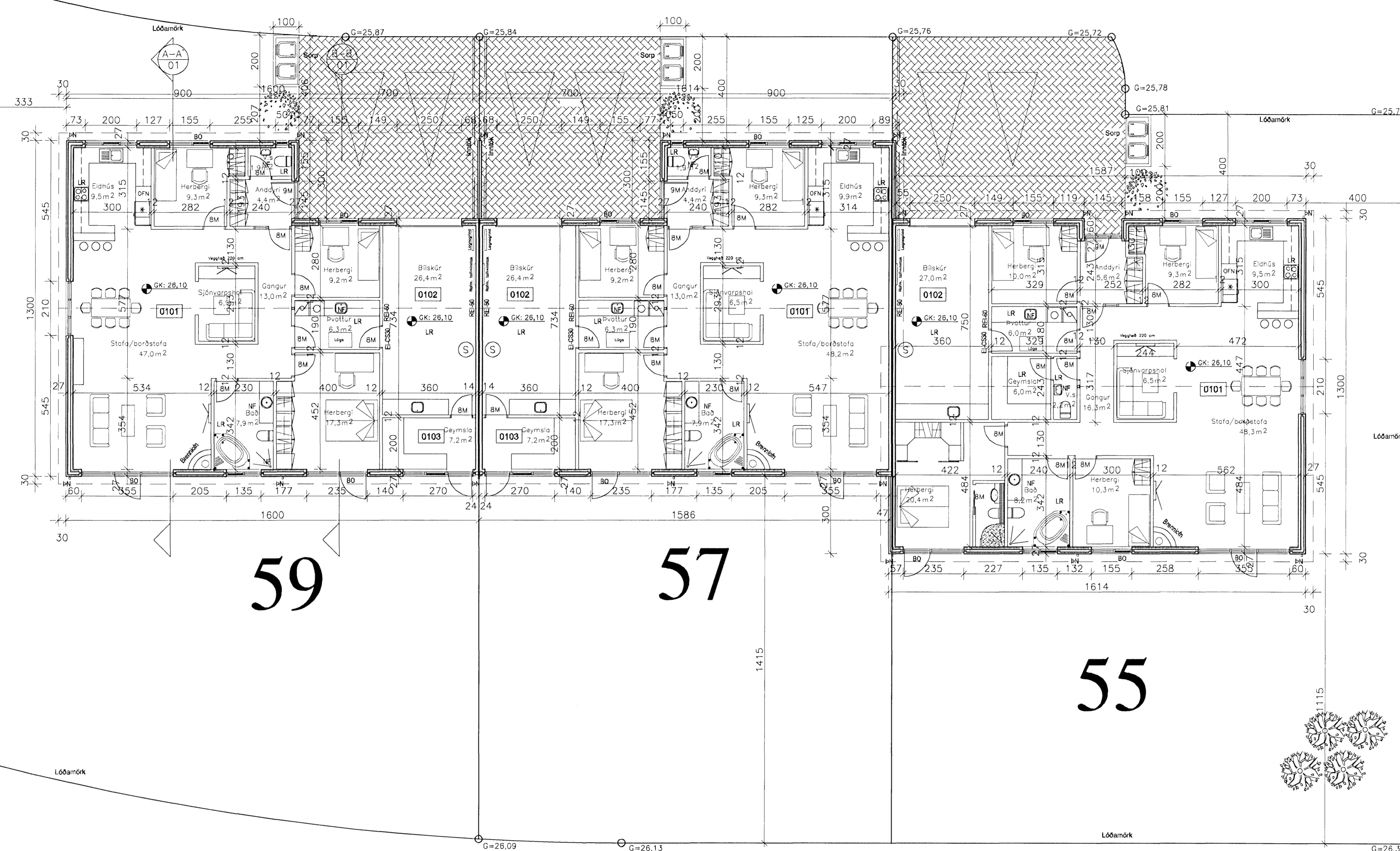
GRUNNMYND 1:100
