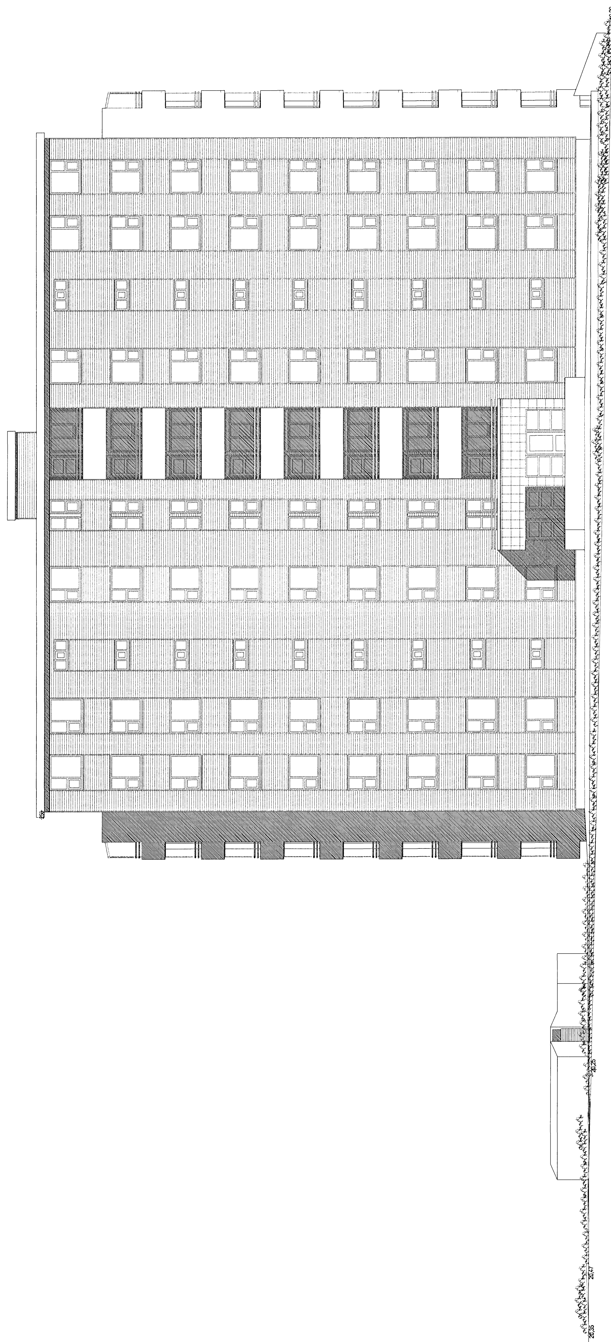
ÚTLIT NORÐUR MKV. 1:100.
