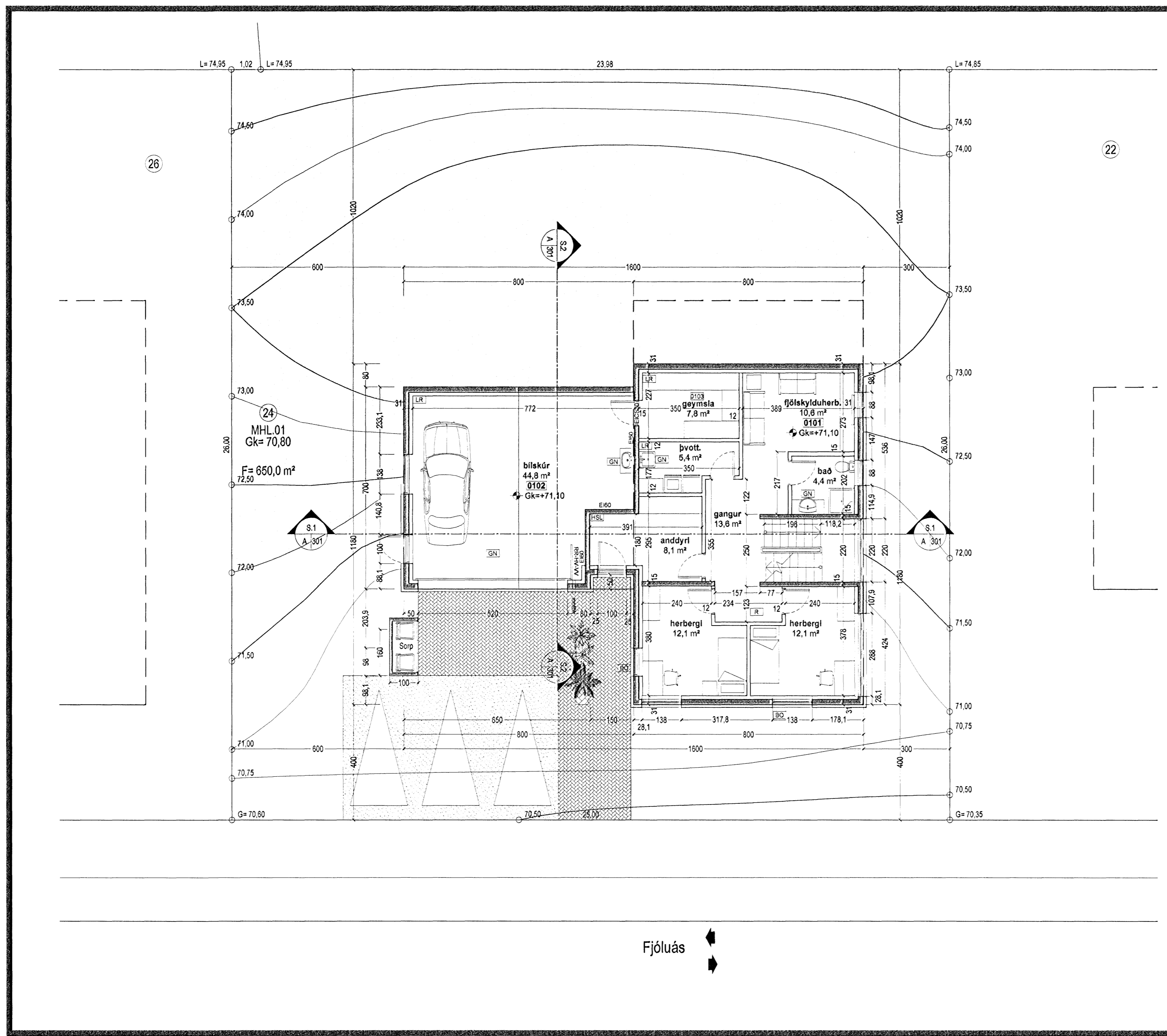
Grunnmynd 1 hæð 1:100
