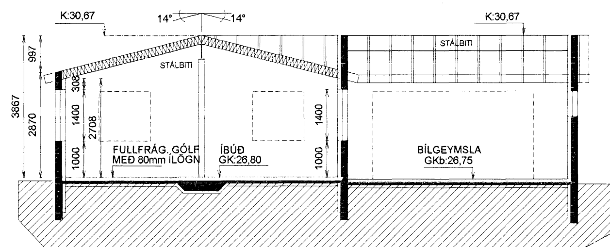
SNÍÐ A-A 1:100
