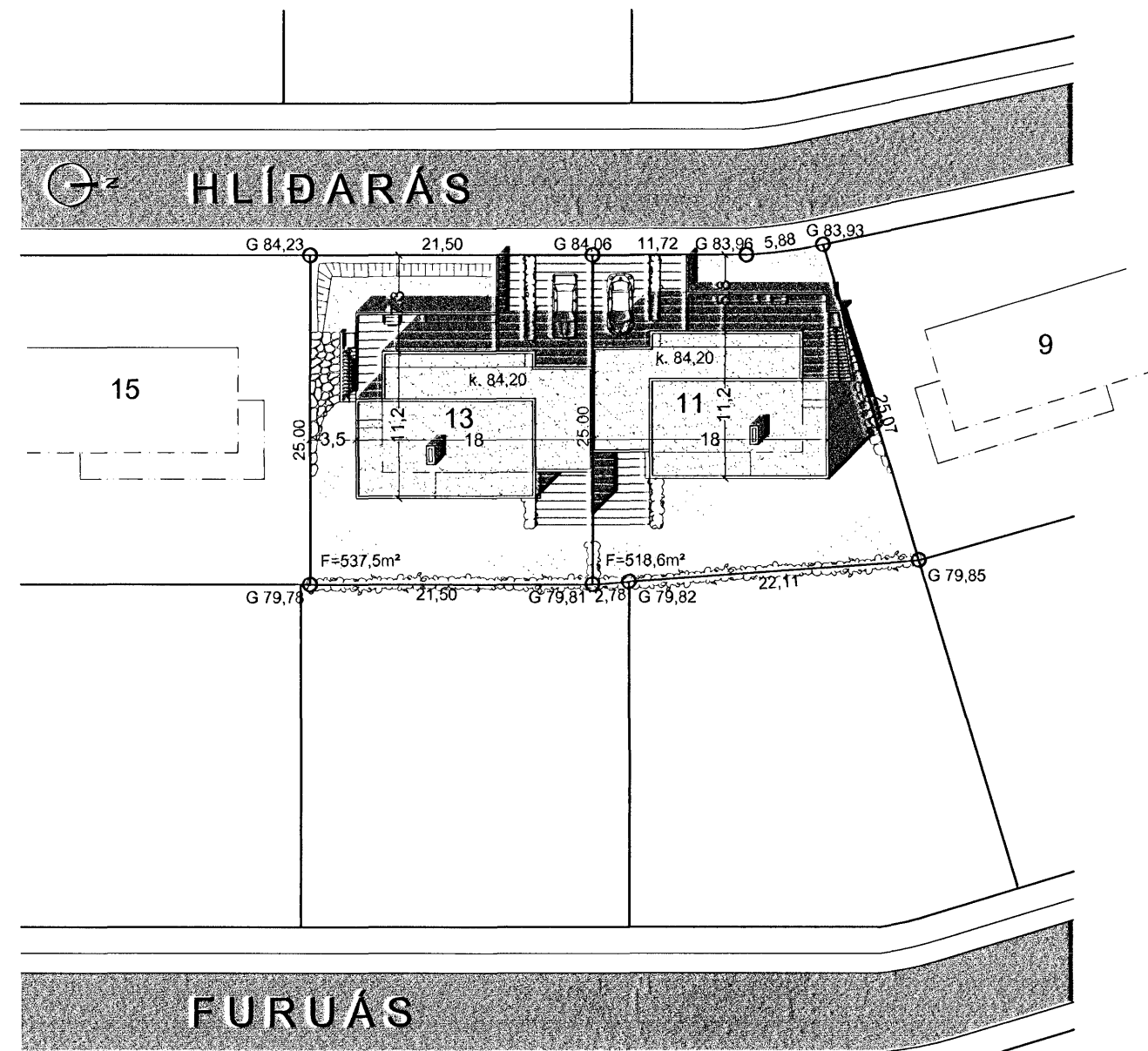
AFSTÖÐUMYND M 1 : 500
