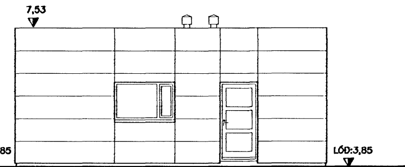
NORDURHLIÐ MKV. 1
