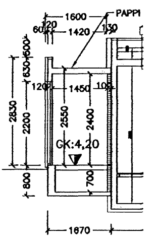
2 SNID MKV. 1
