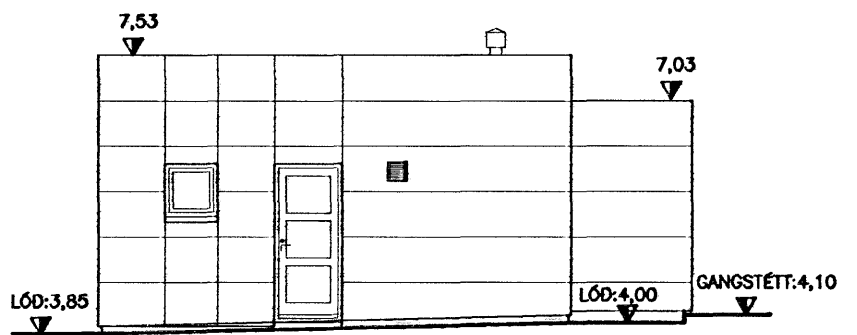
VESTURHLIÐ MKV. 1
