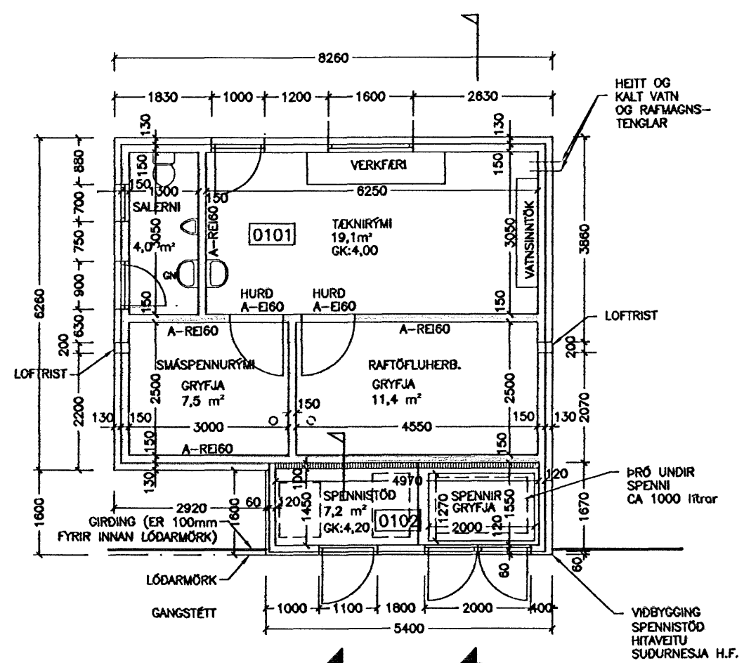
GRUNNMYND MKV. 1
