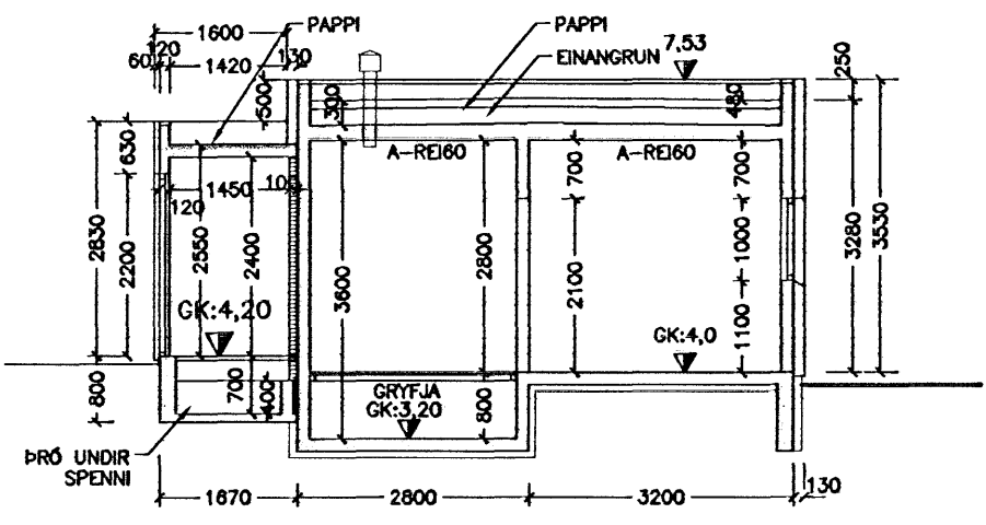
1 SNID MKV. 1
