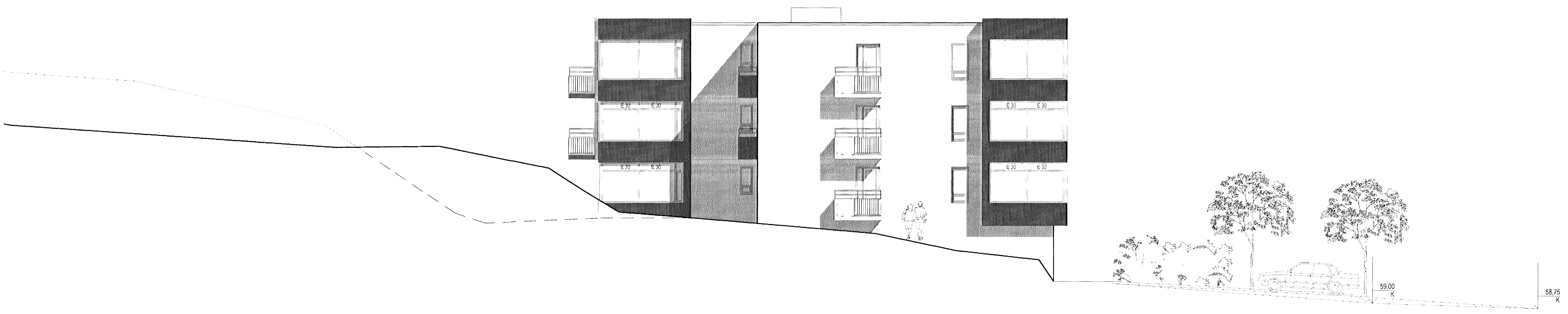
ÚTLIT 1:100 ÚTLIT SUÐUR
