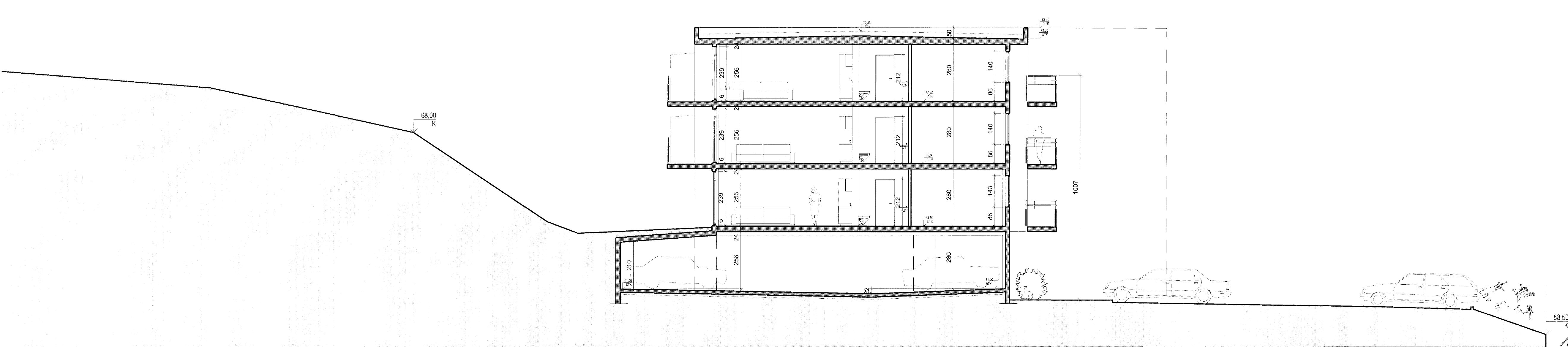
SNEIÐING 1:100 Sneiðing A-A
