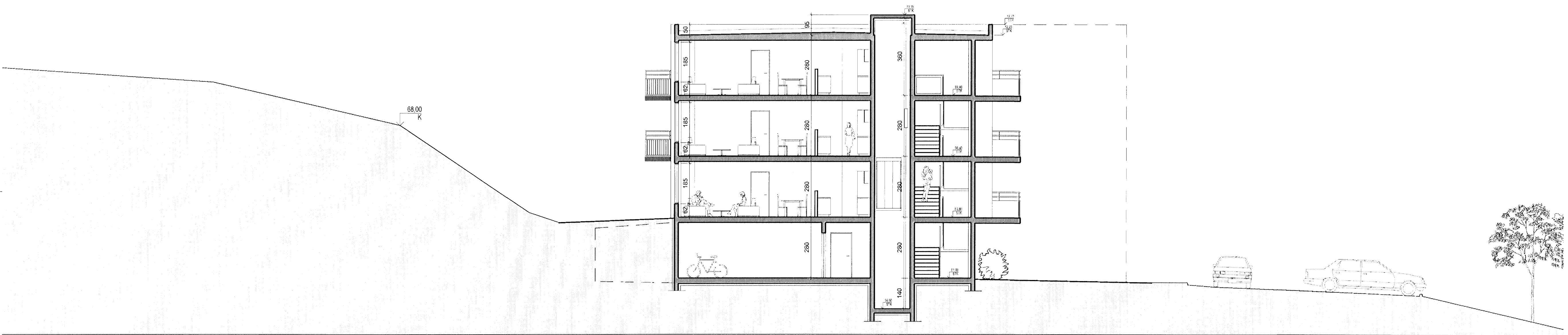
SNEIÐING 1:100 Sneiðing B-B
