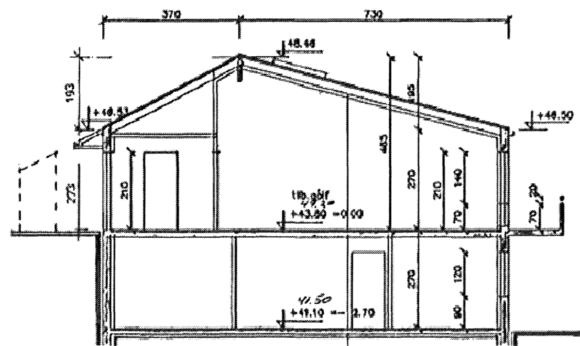
SNOMYND A-A KLUKKUBERG 2
