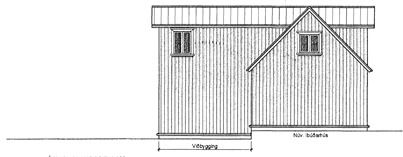
ÚTLIT VESTURGAFL 1:100
