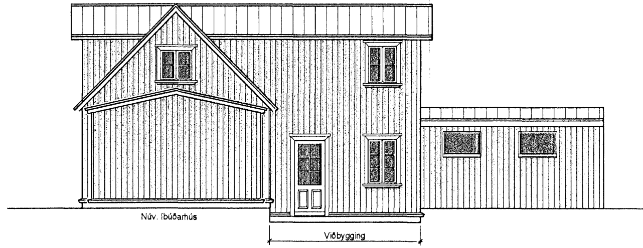
ÚTLIT AUSTURGAFL 1:100
