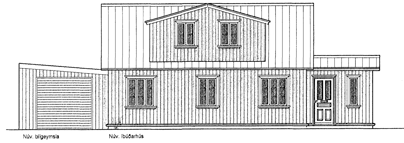
ÚTLIT SUÐURHLIÐ 1:100
