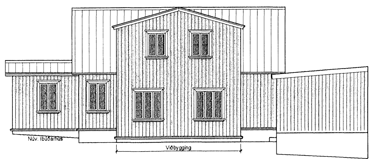
ÚTLIT NORÐURHLIÐ 1:100
