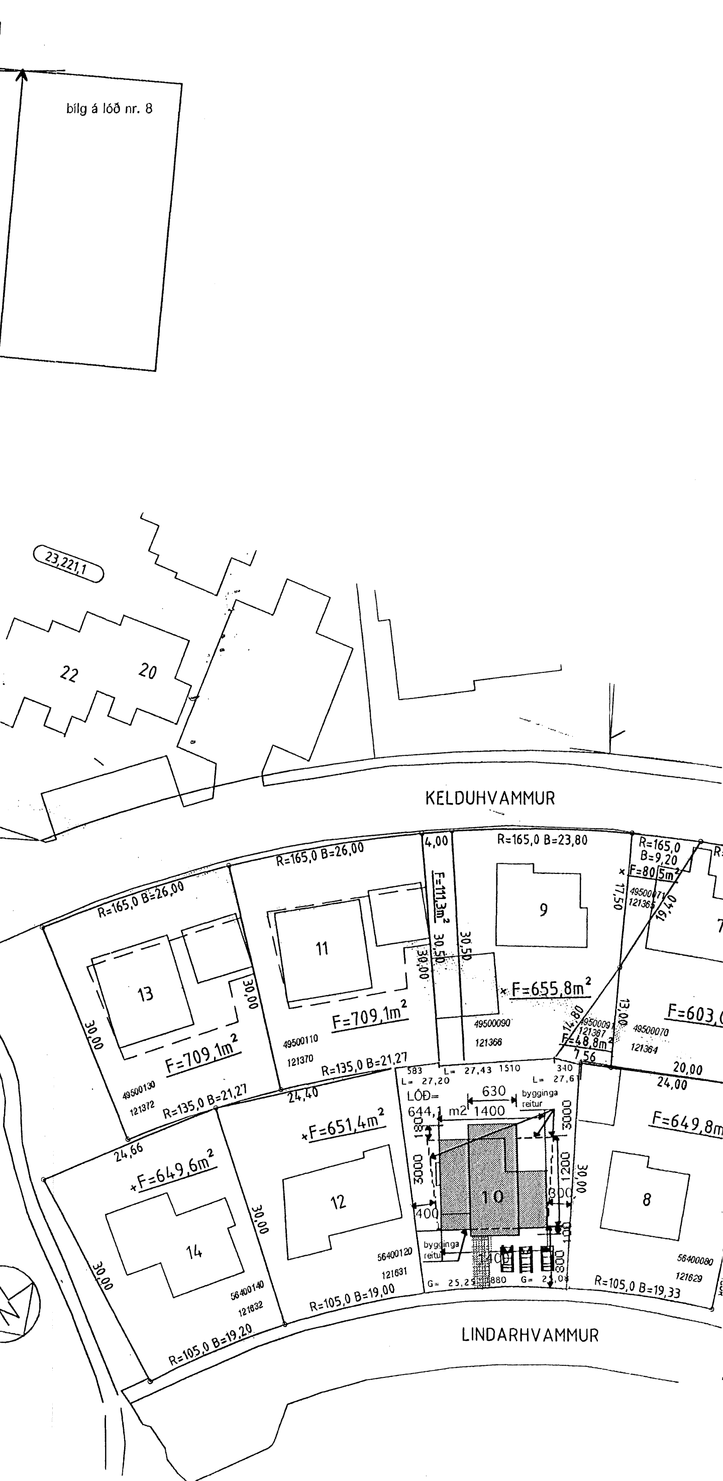
AFSTÖÐUMYND 1:500
