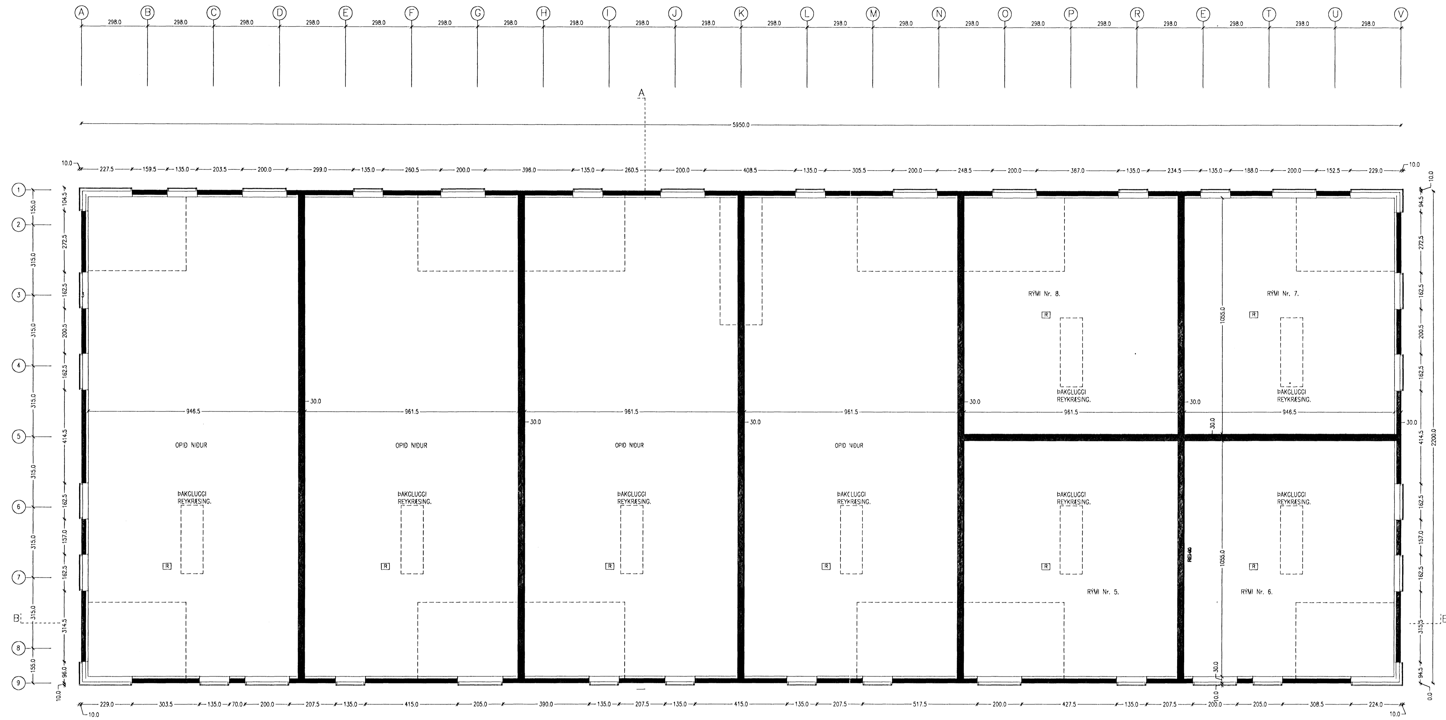
GRUNNMÝND 2 HÆÐAR 1:100
