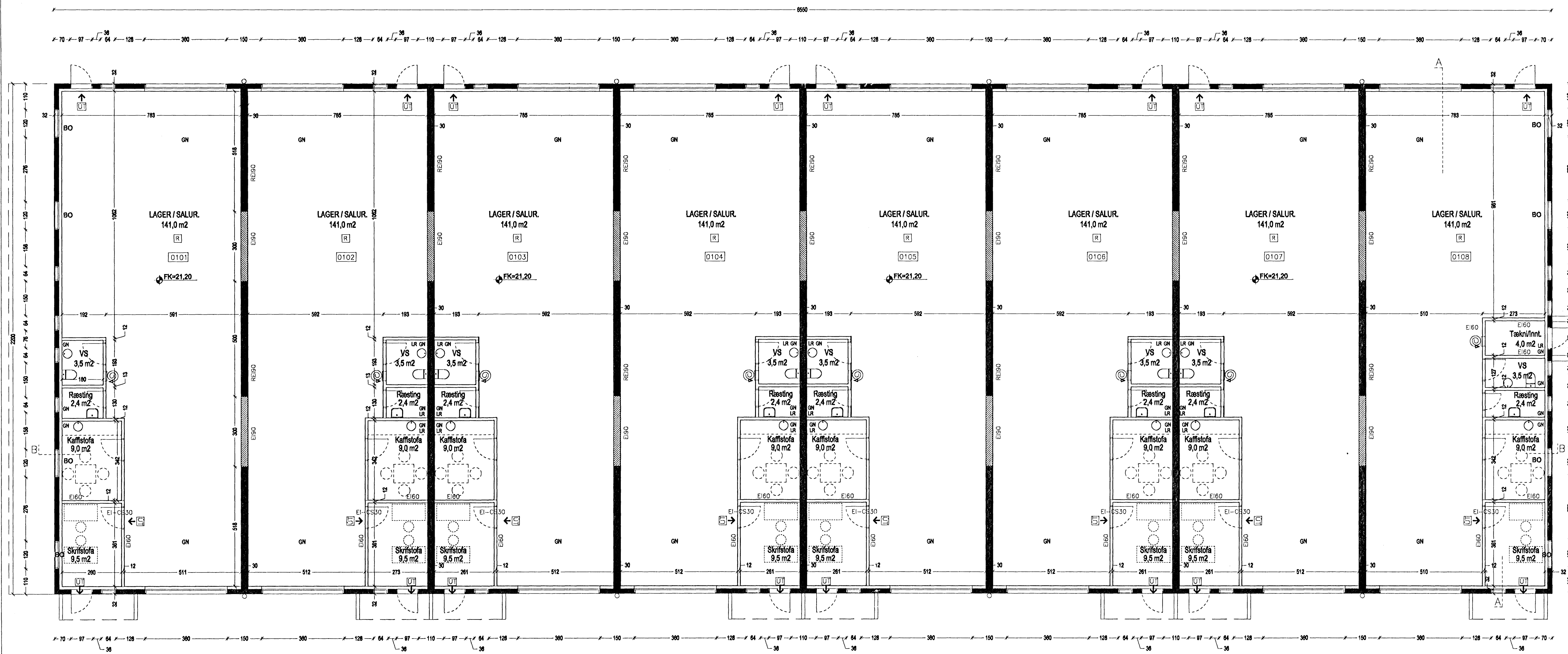
GRUNNMYND 1 HÆÐAR 1:100
