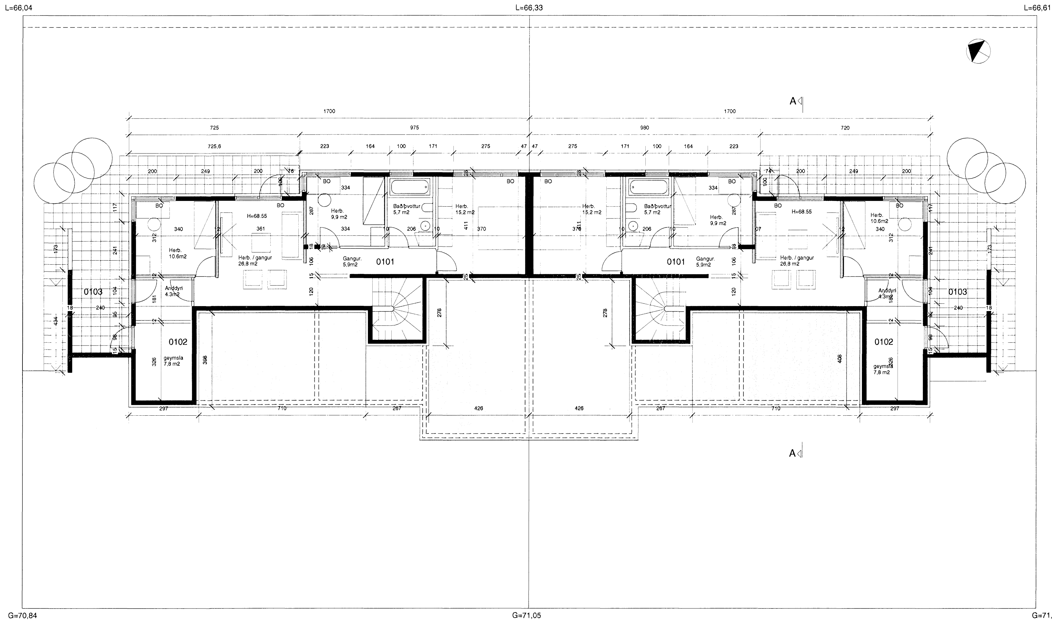
GRUNNMYND 1. HÆÐ
