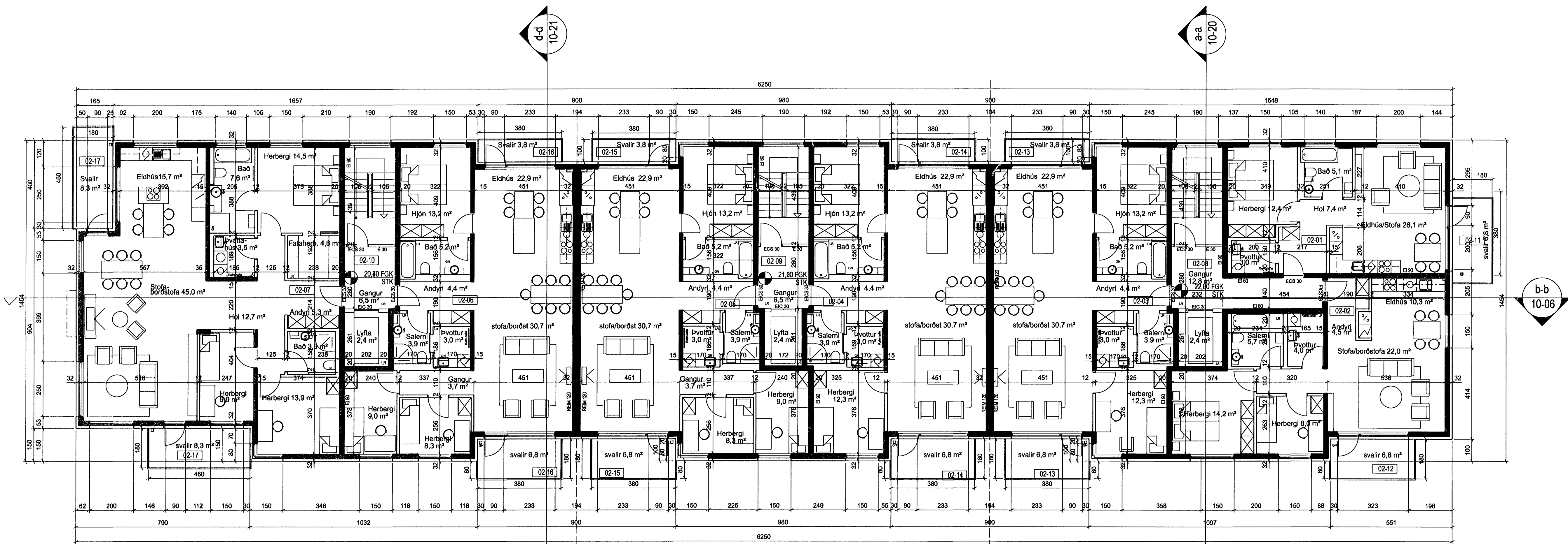
GRUNNMYND 2. HÆÐ 1:100
