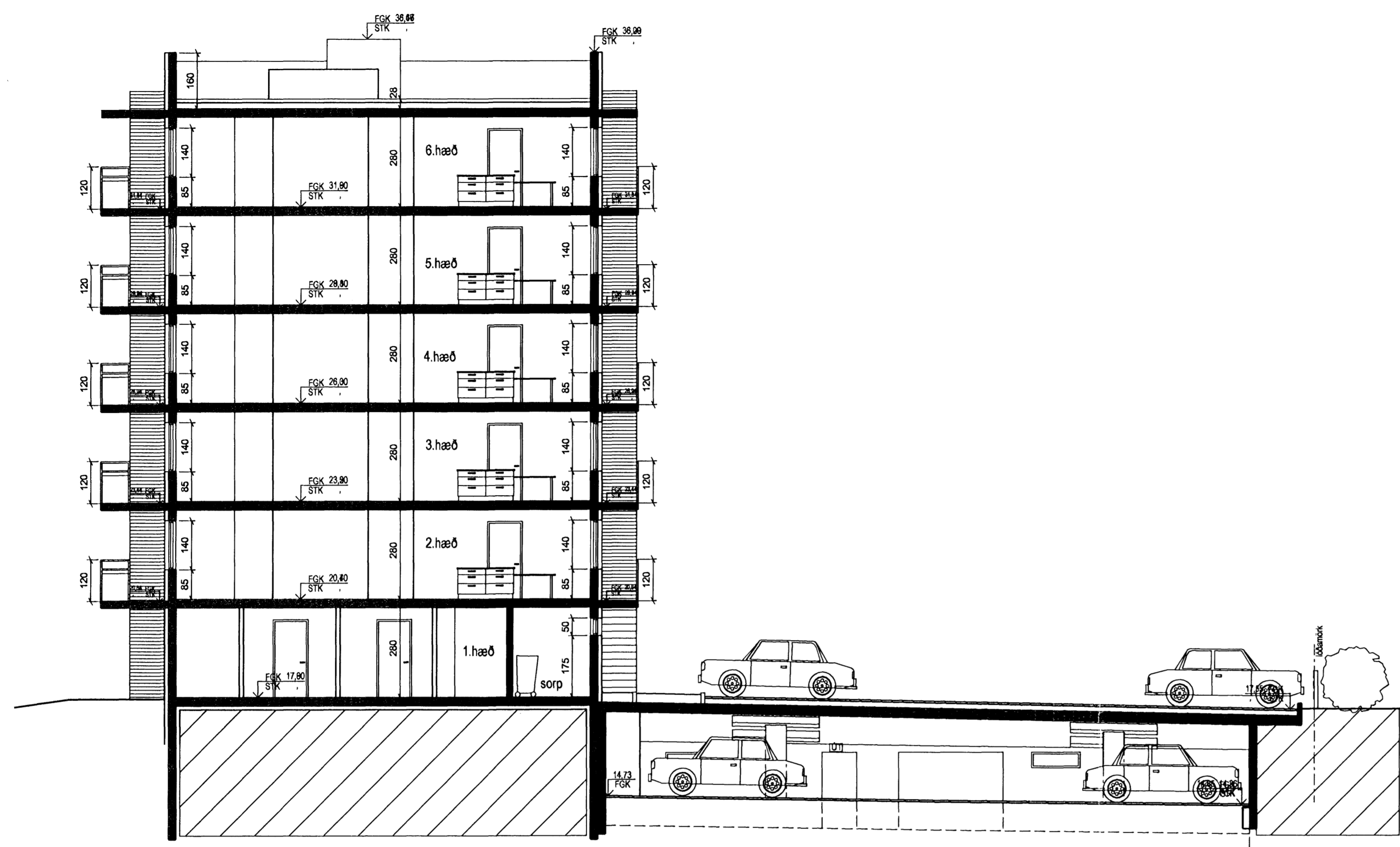
SNEIÐING 1:100 sníð D-D
