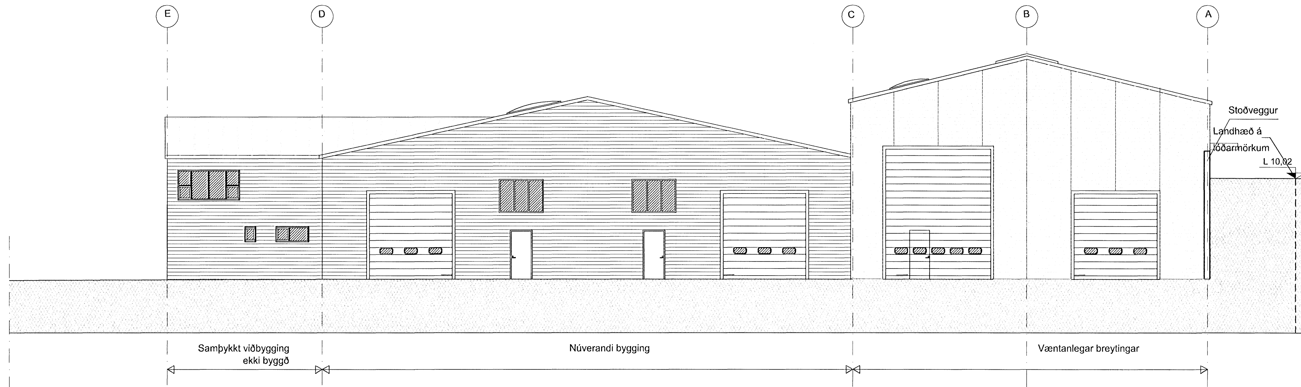
Útlit suðvestur, mkv. 1:100
