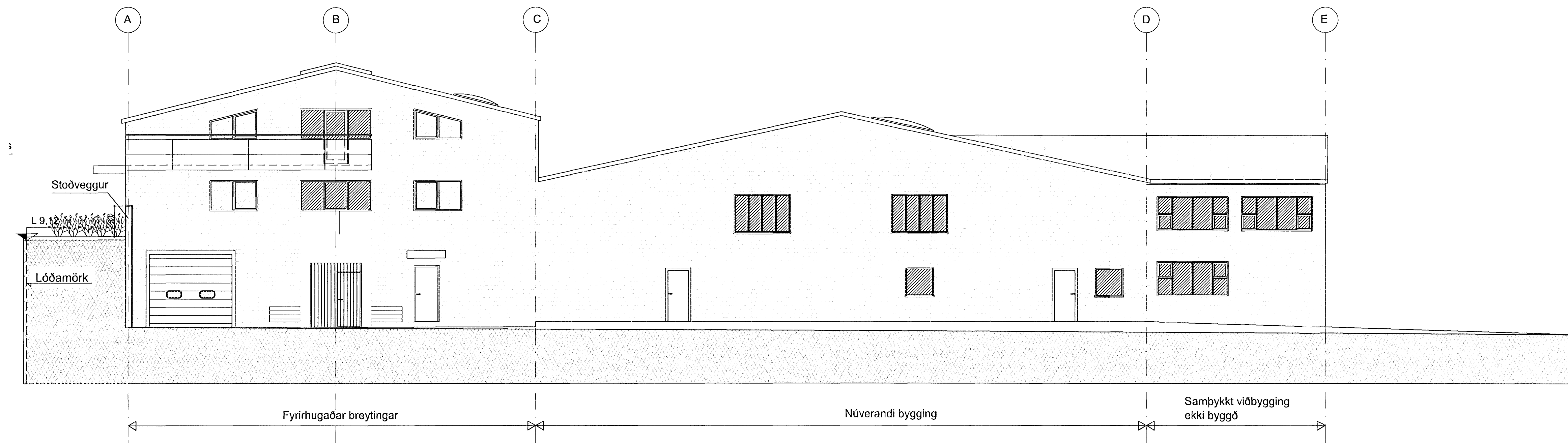
Útlit norðaustur, mkv. 1:100
