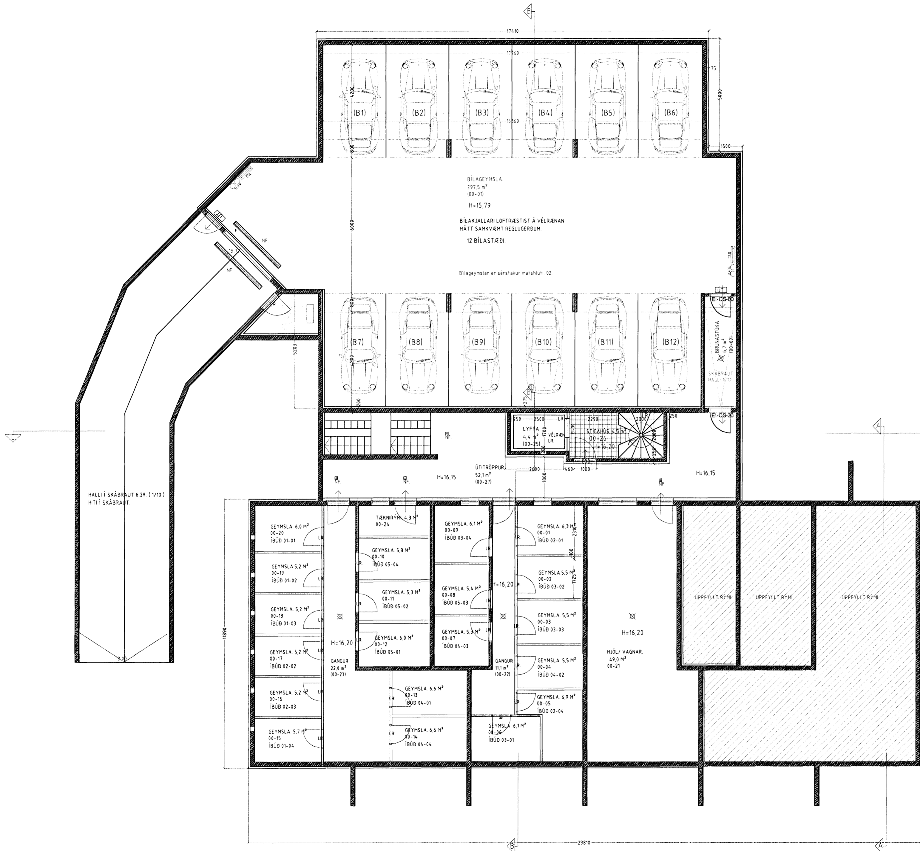
GRUNNMYND KJALLARA, MKV. 1:100.
