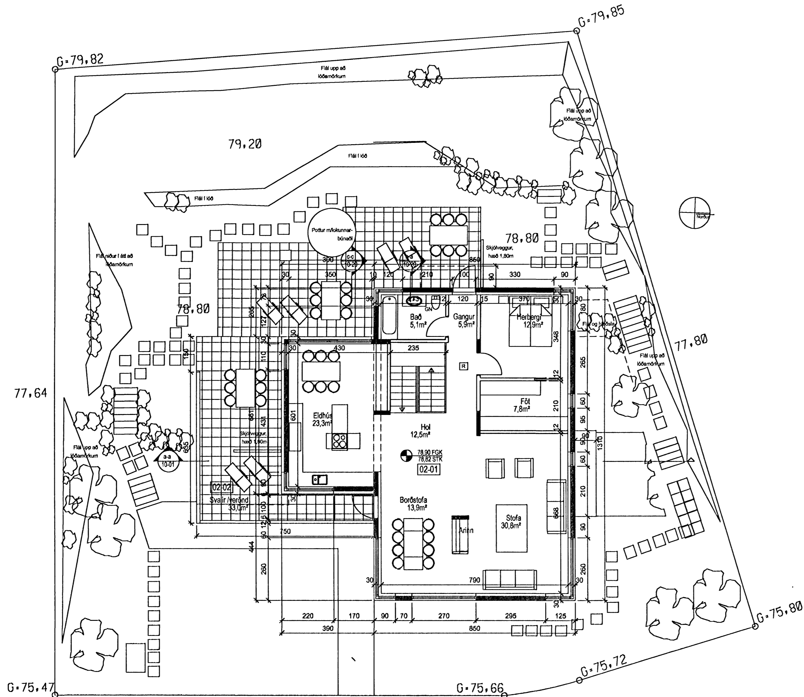
Grunnmynd 2.hæð 1:100
