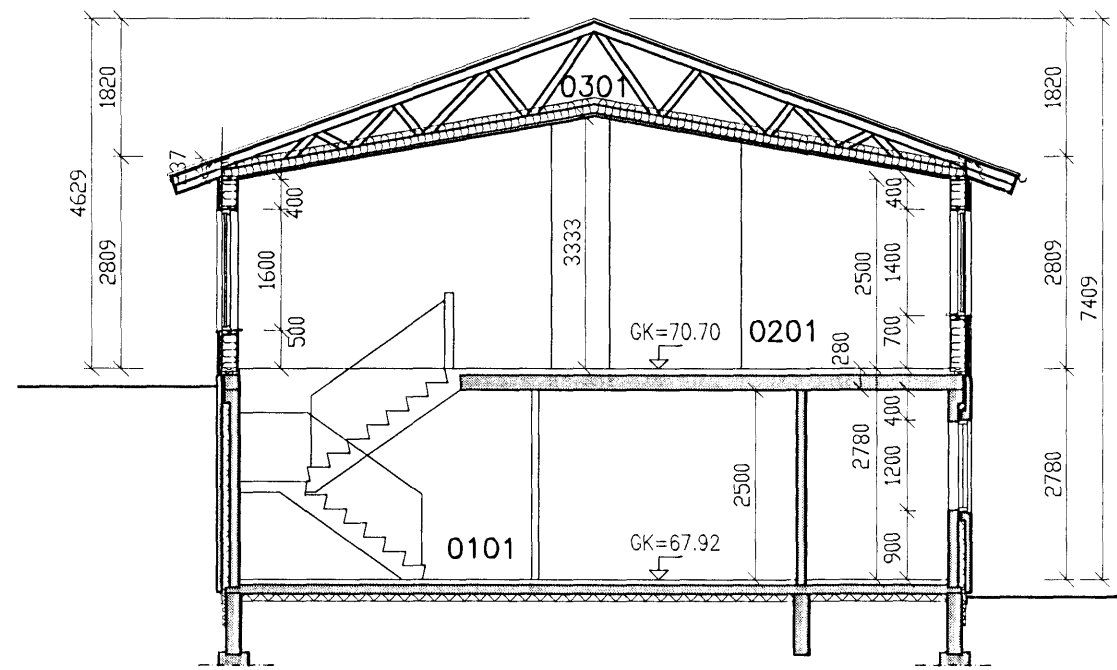
SNID 1-1 1:100
