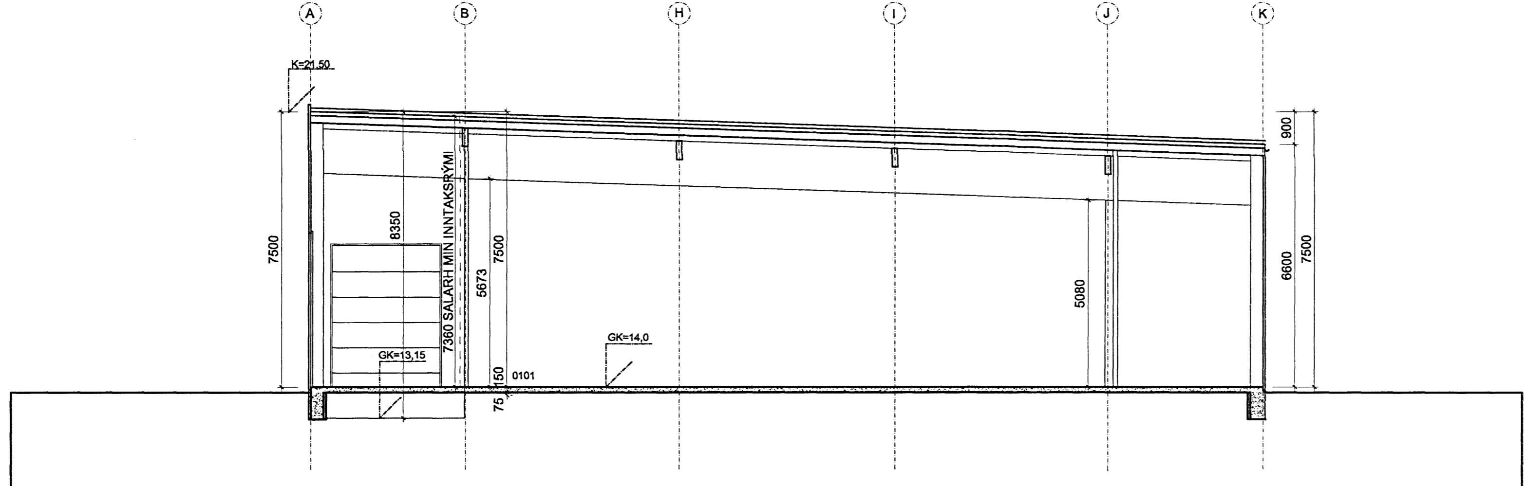
SNEIÐING B-B, M: 1/100,
