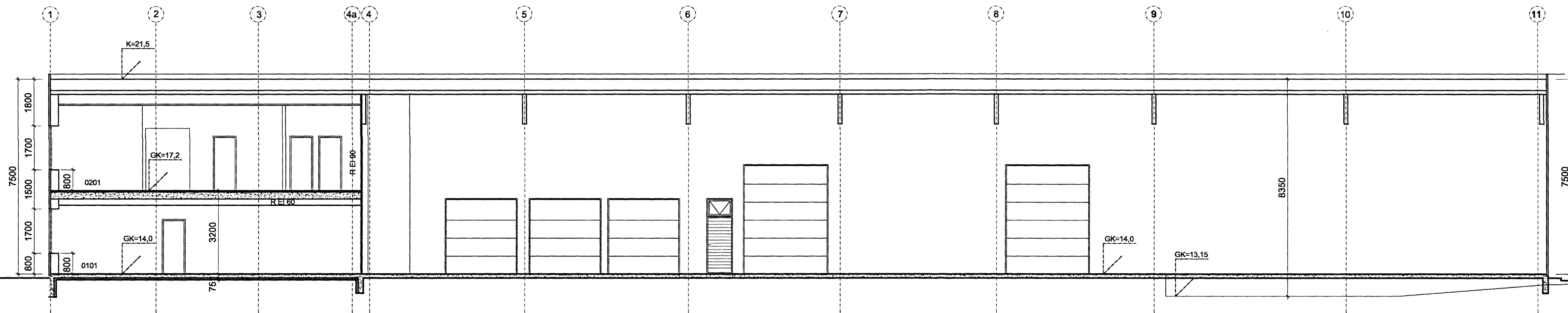
SNEIÐING A-A, M: 1/100,
