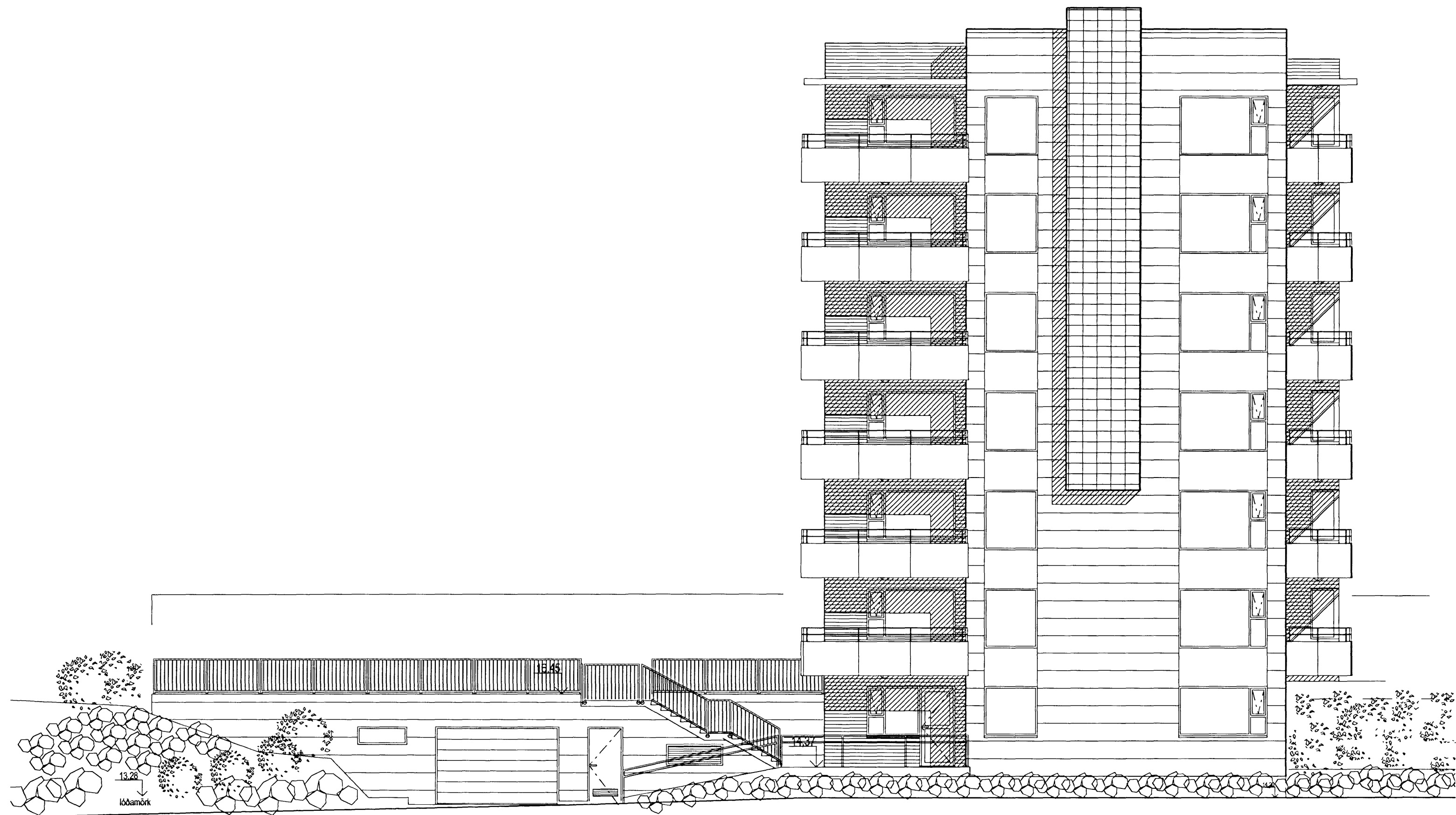
ÚTLIT 1:100 norð vestur hlíð
