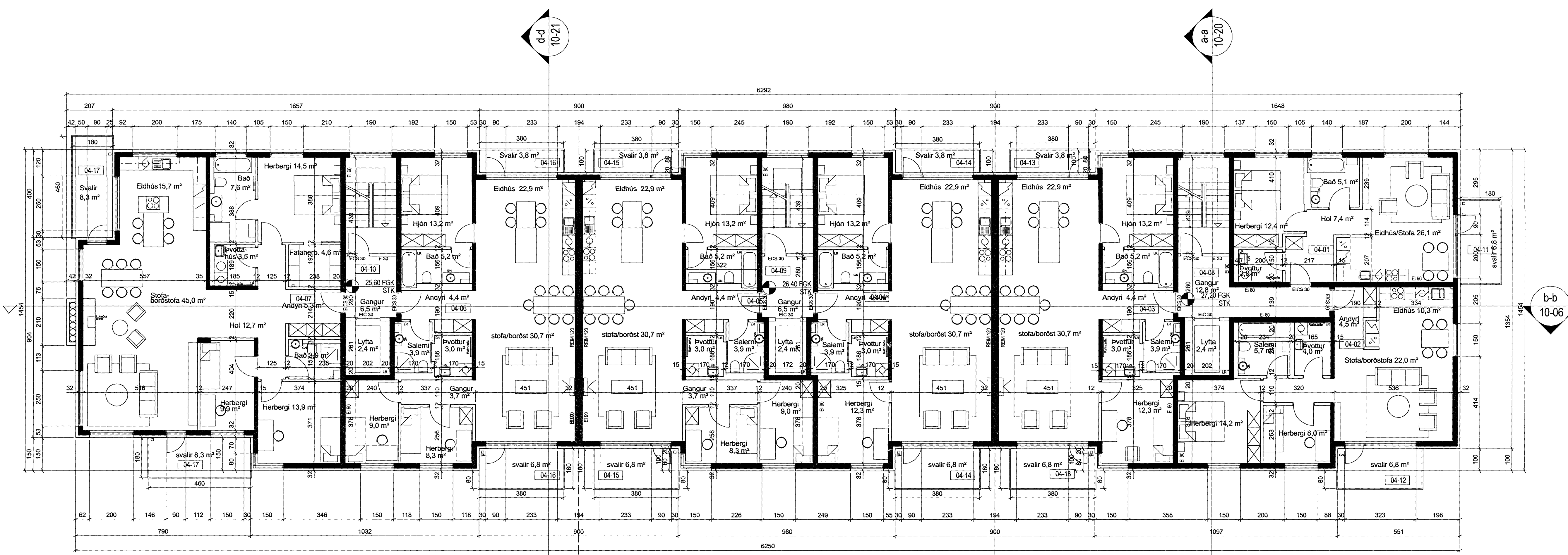
GRUNNMYND 4. HÆÐ 1:100
