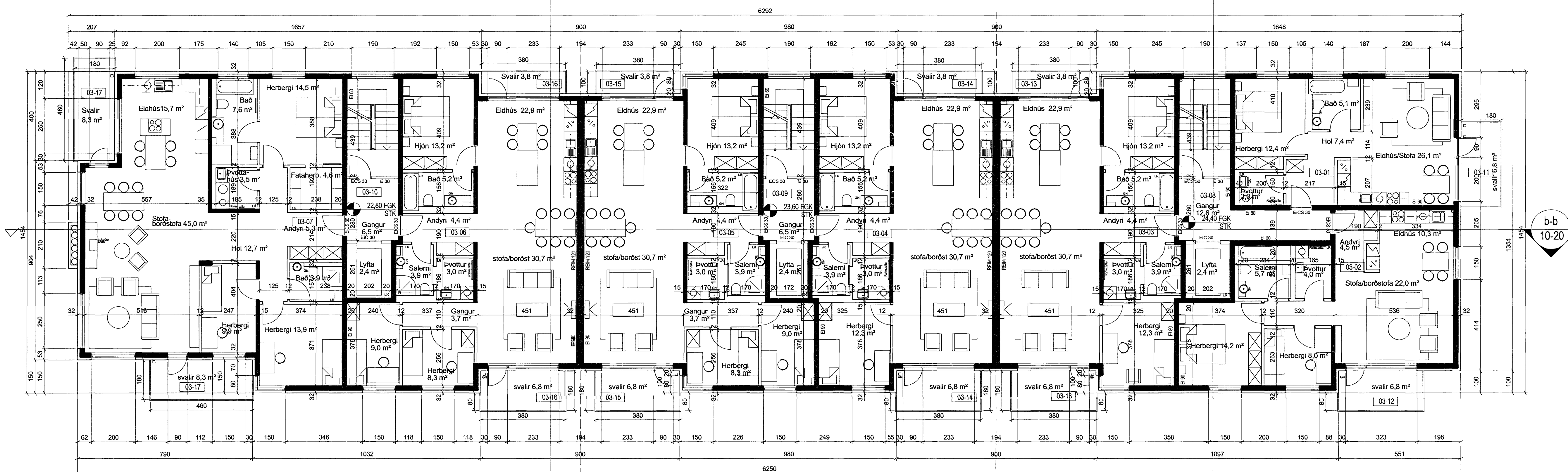
GRUNNMYND 2. HÆÐ 1:100
