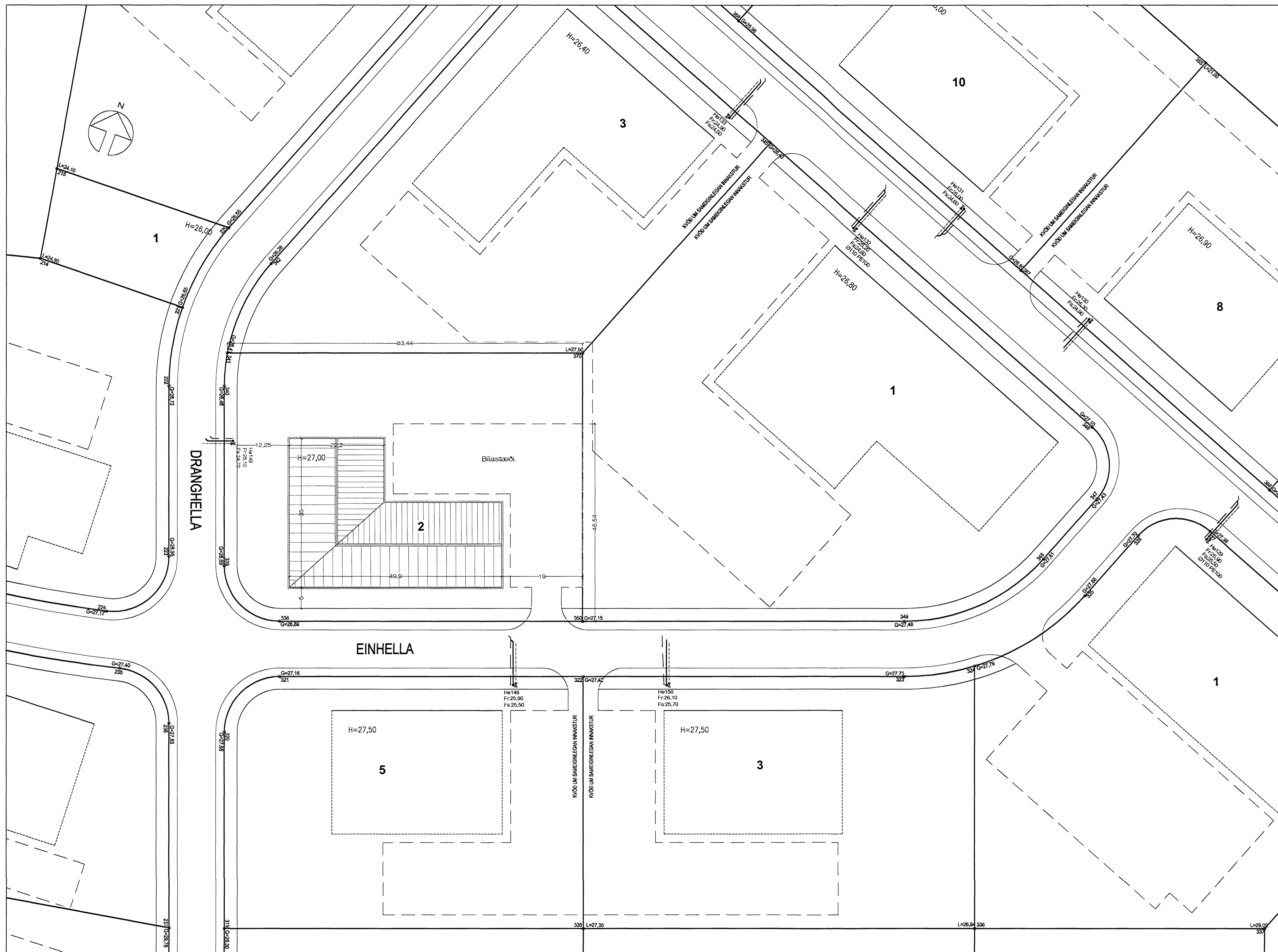
Afstöðumynd. 1:500
