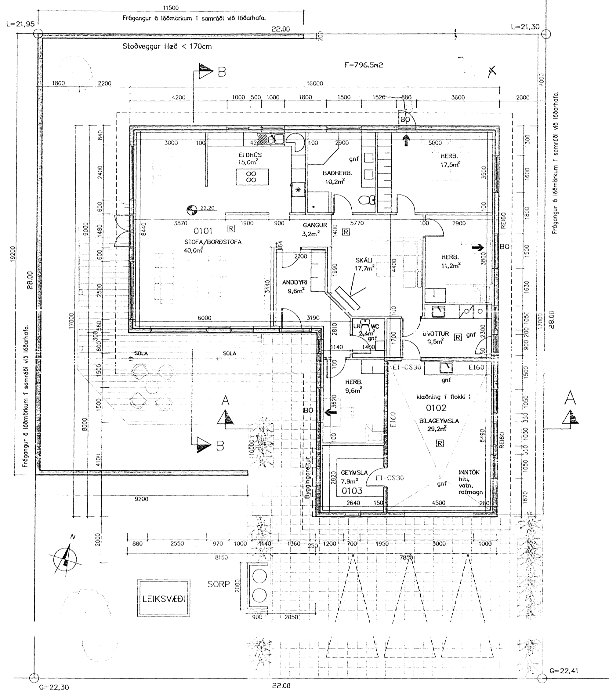
GRUNNMYND 1:100
