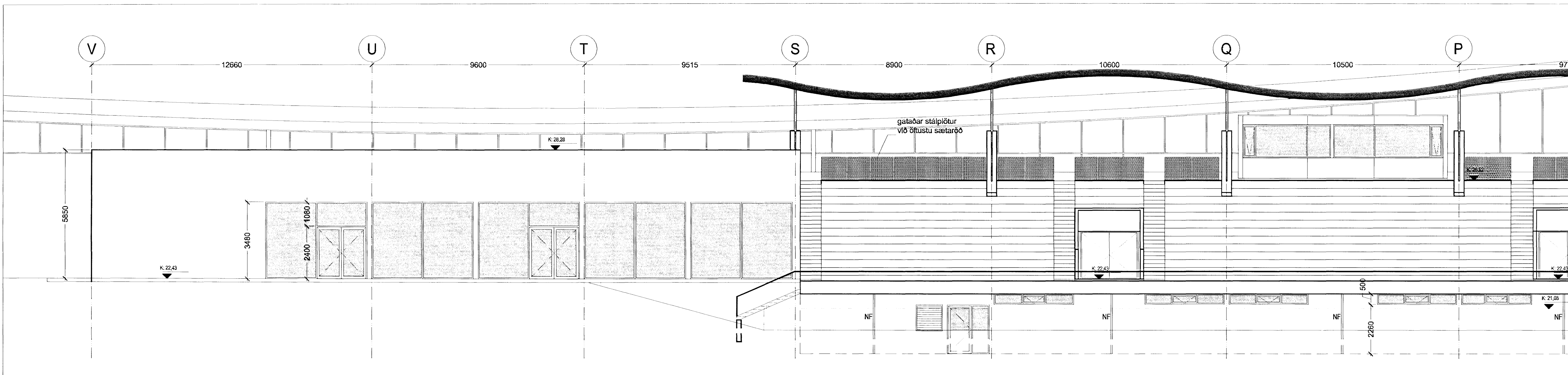
NORÐURHLIÐ D-BYGGINGAR í mkv. 1:100
