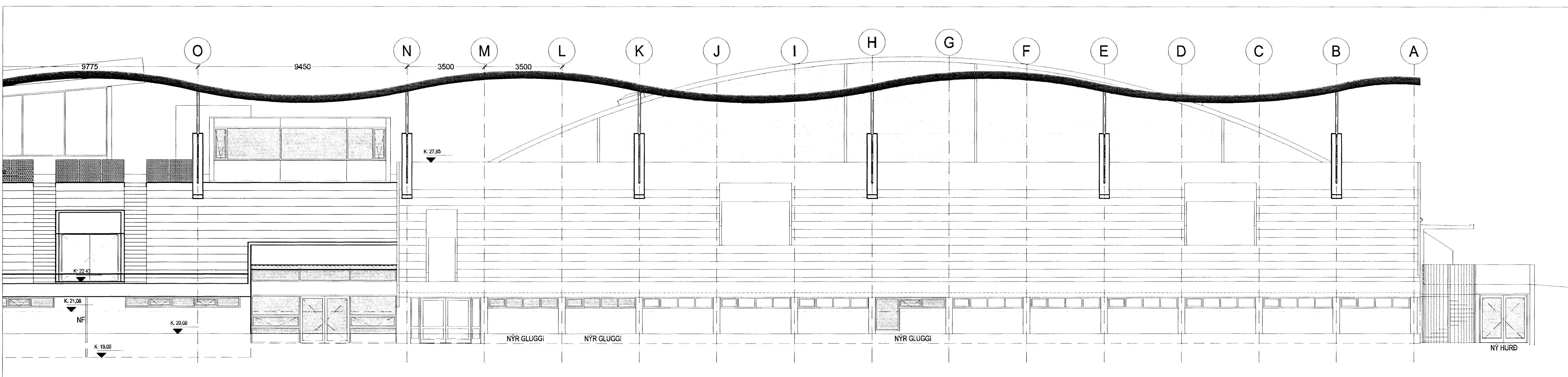
NORÐURHLIÐ D OG A-BYGGINGAR í mkv. 1:100
