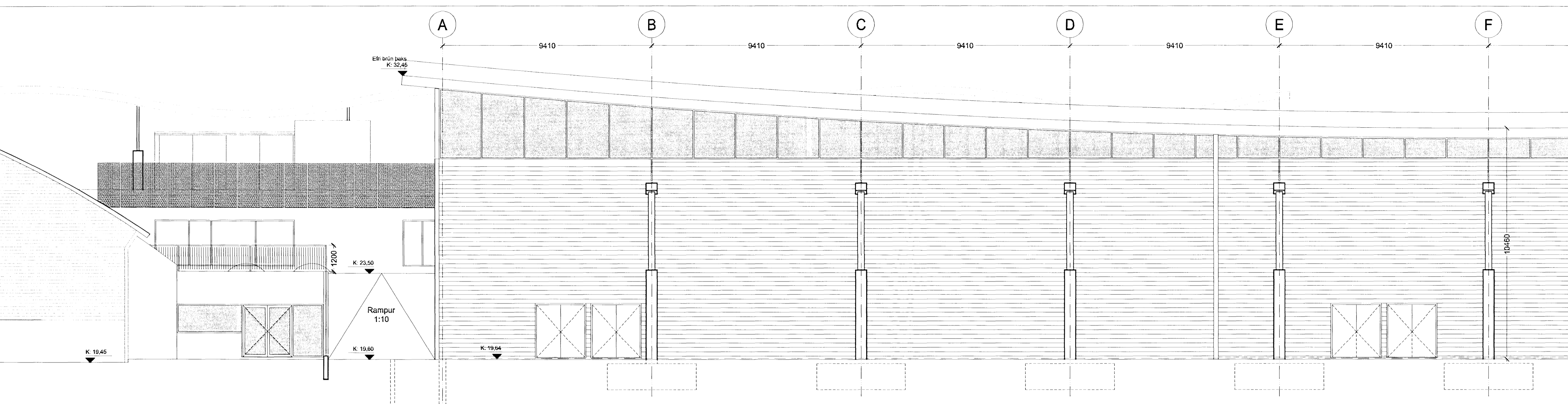
SUBURHLIÐ E-BYGGINGAR í mkv. 1:100
