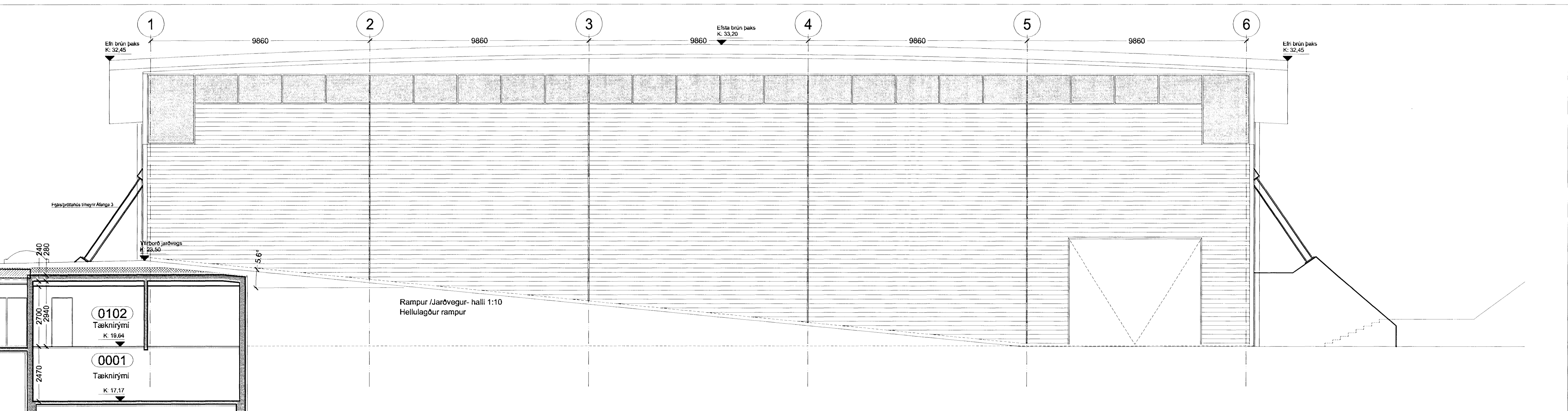
VESTURHLIÐ E-BYGGINGAR í mkv. 1:100
