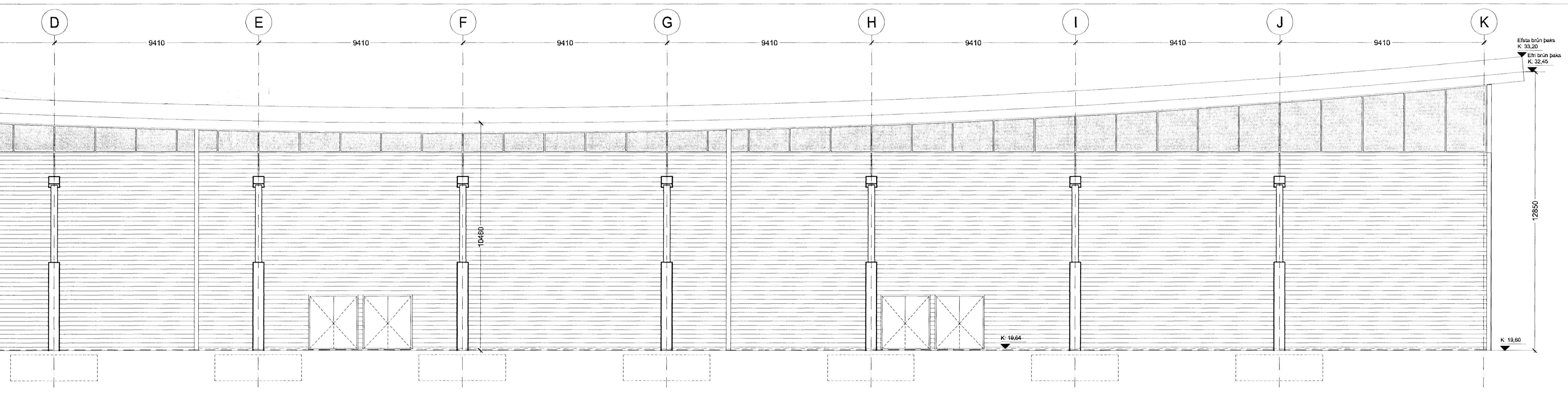
SUBURHLIÐ E-BYGGINGAR í mkv. 1:100
