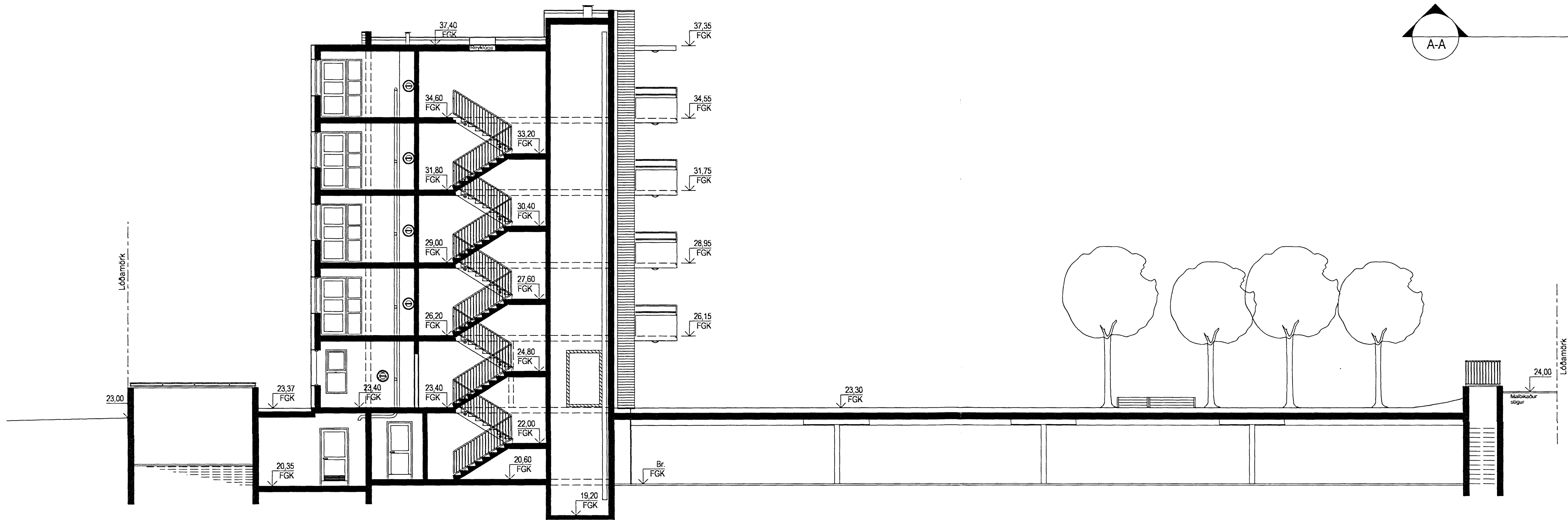
B-B SNEIDING 1:100
