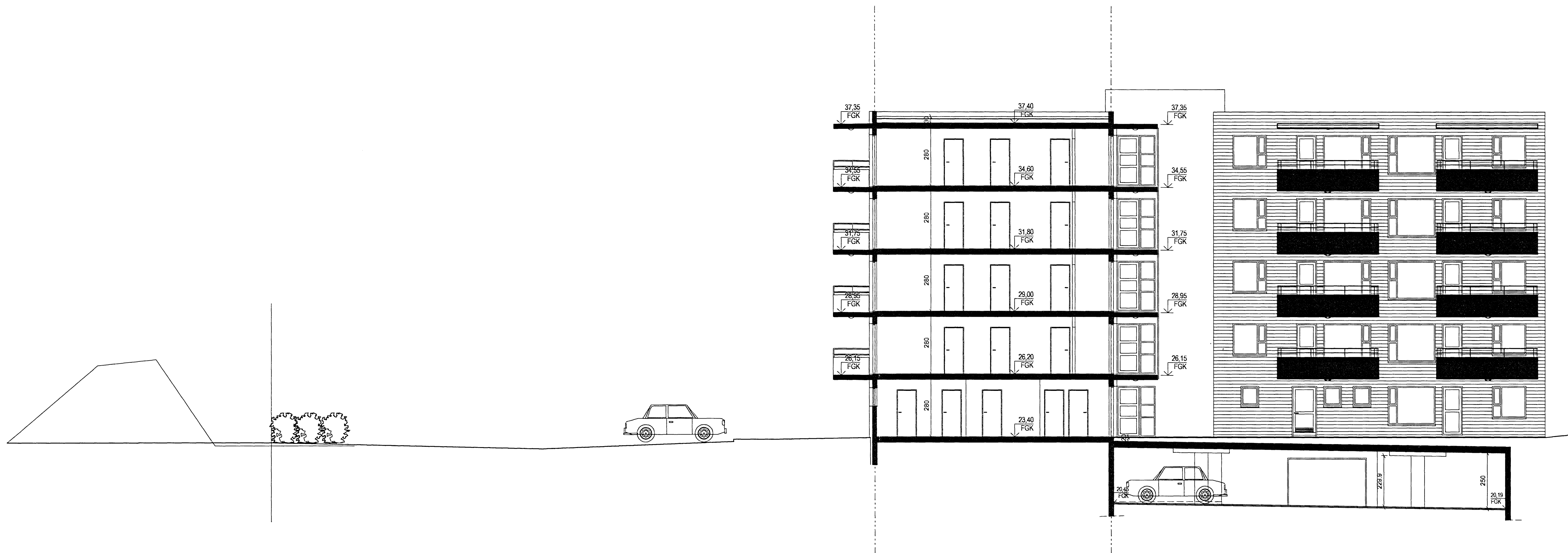
A-A SNEIDING 1:100
