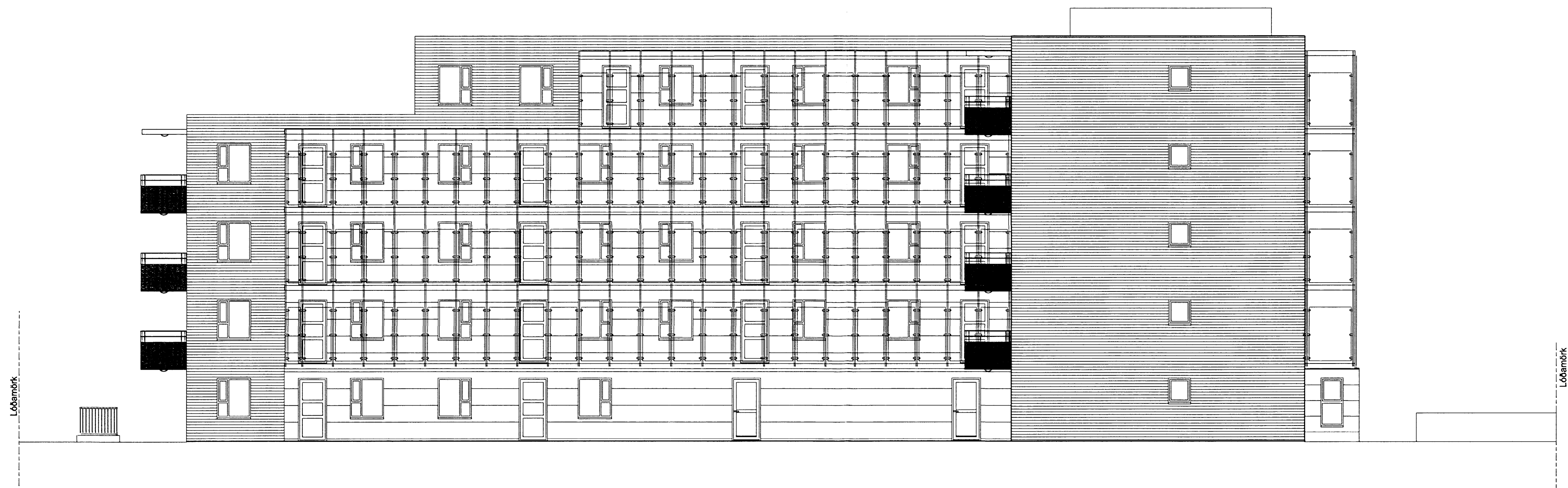
ÚTLIT 1:100 Norður
