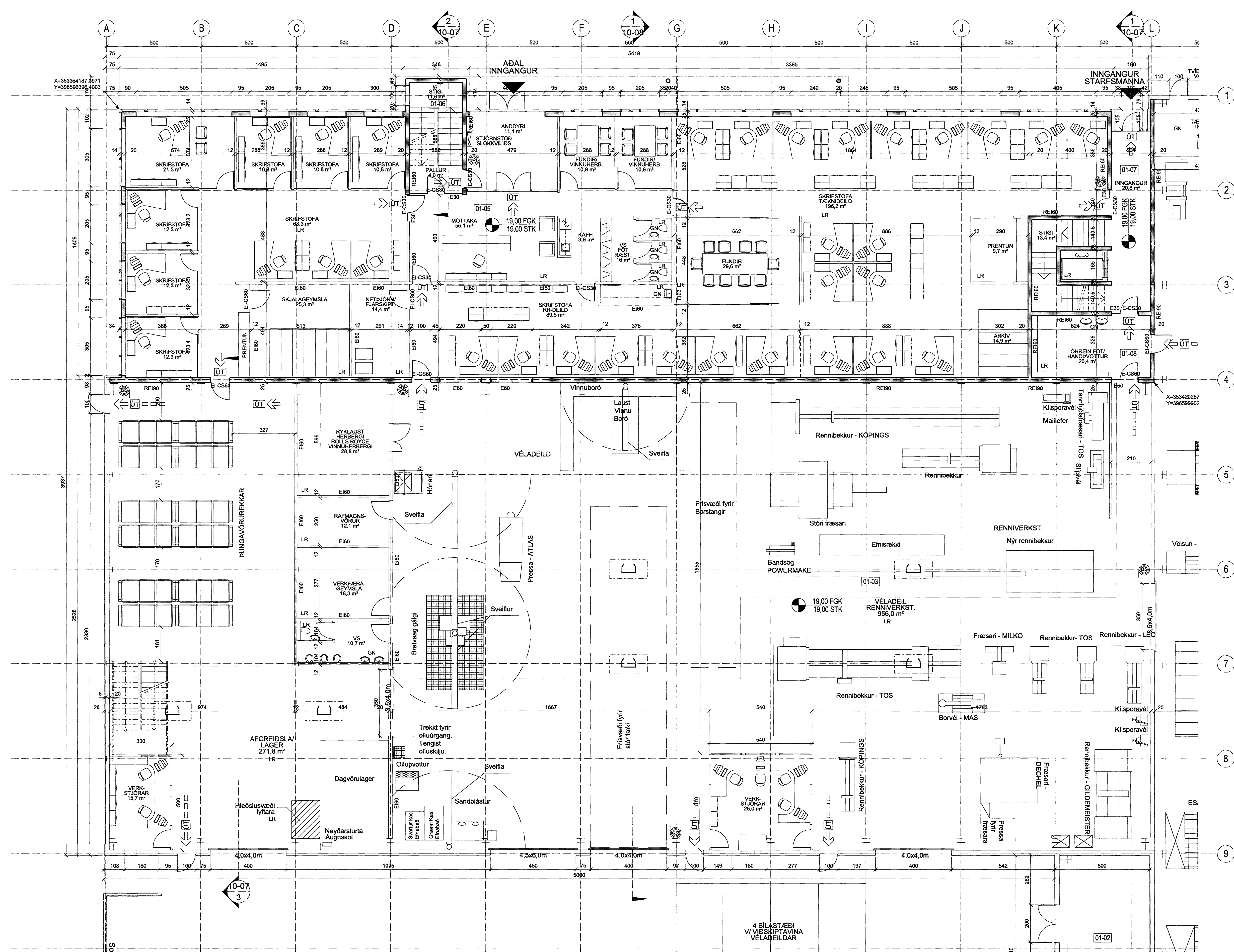
1 GRUNNMYND 1.HÆÐ (hluti) 1:100 Skrifstofur, tækniheilid, afgreiðsla, vélaheild, renniverkstæði
