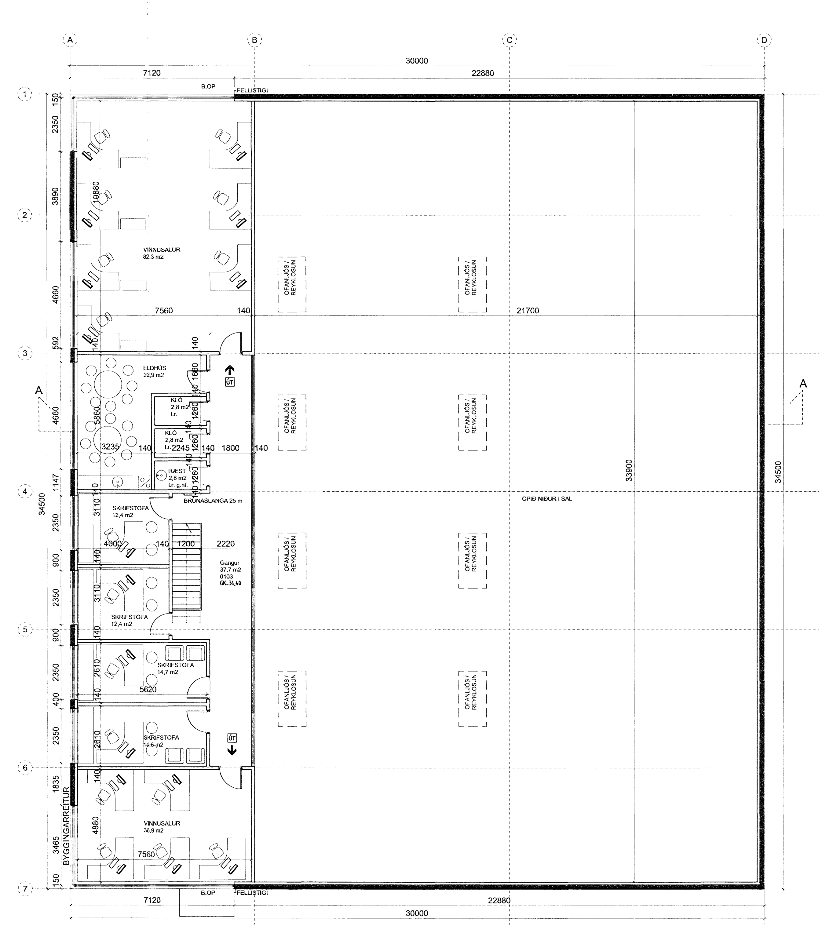
GRUNNMYND MILLIPALLUR 1/100
