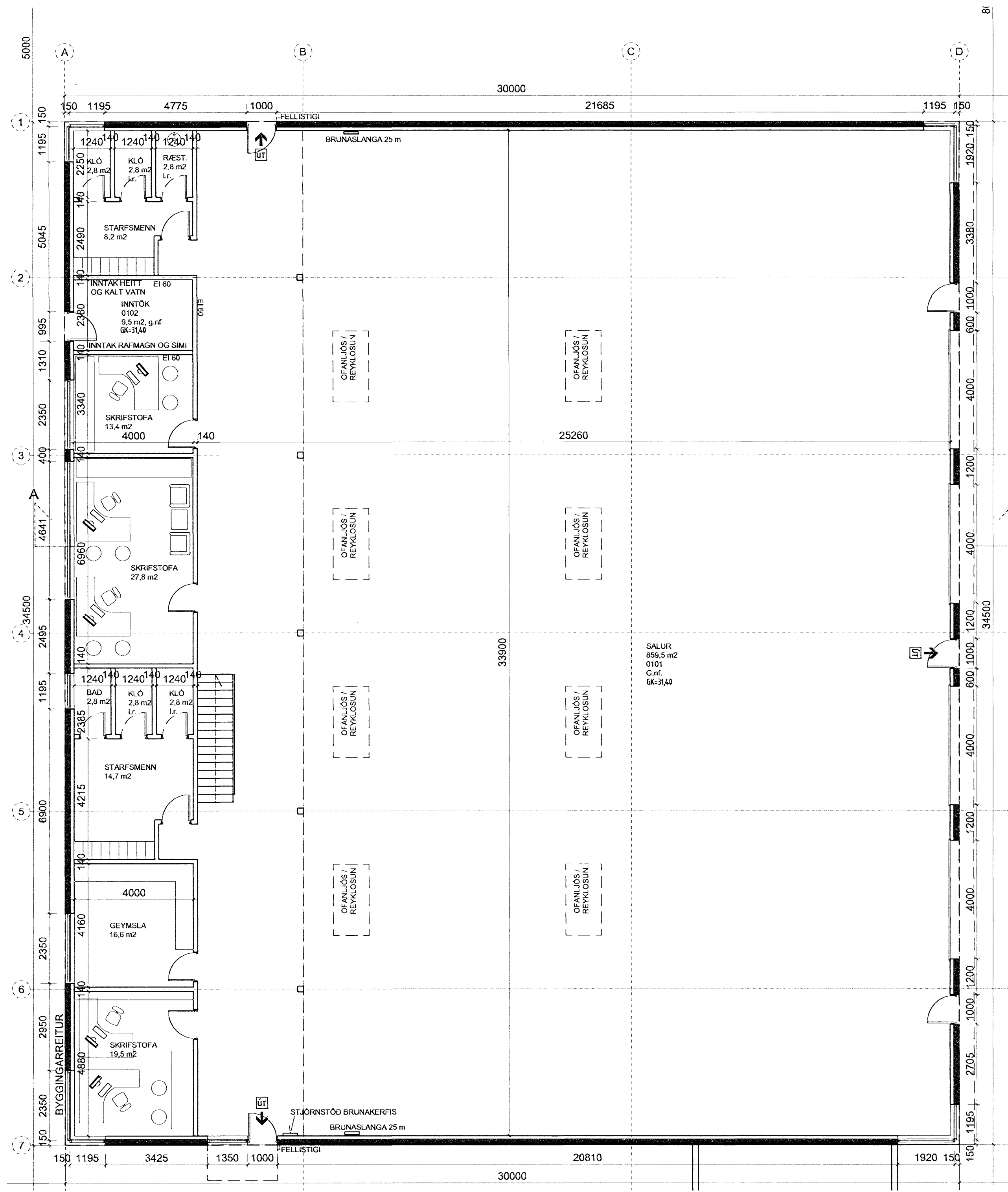
GRUNNMYND 1. HÆÐ 1/100
