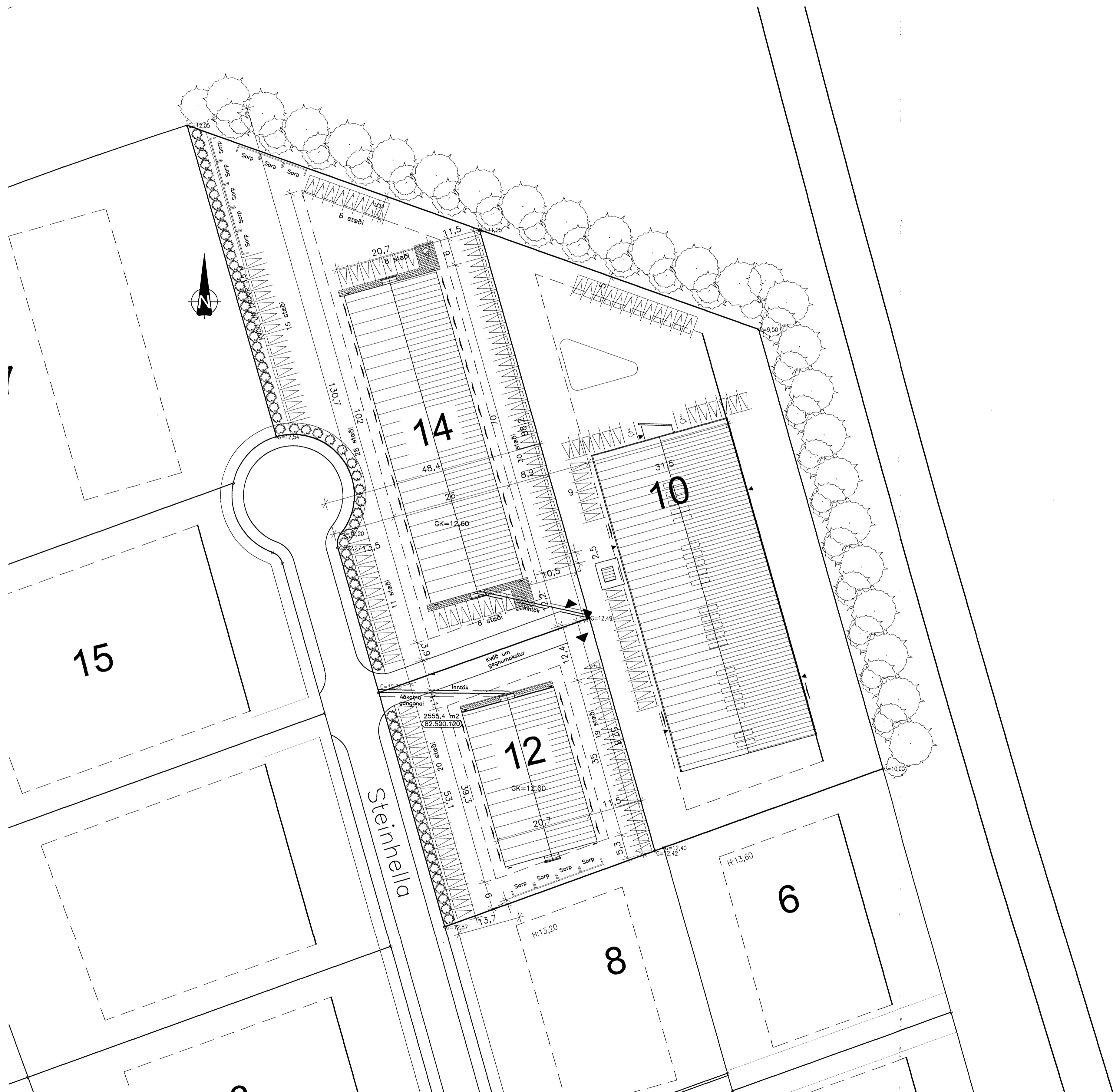
AFSTÖÐUMYND 1:500
