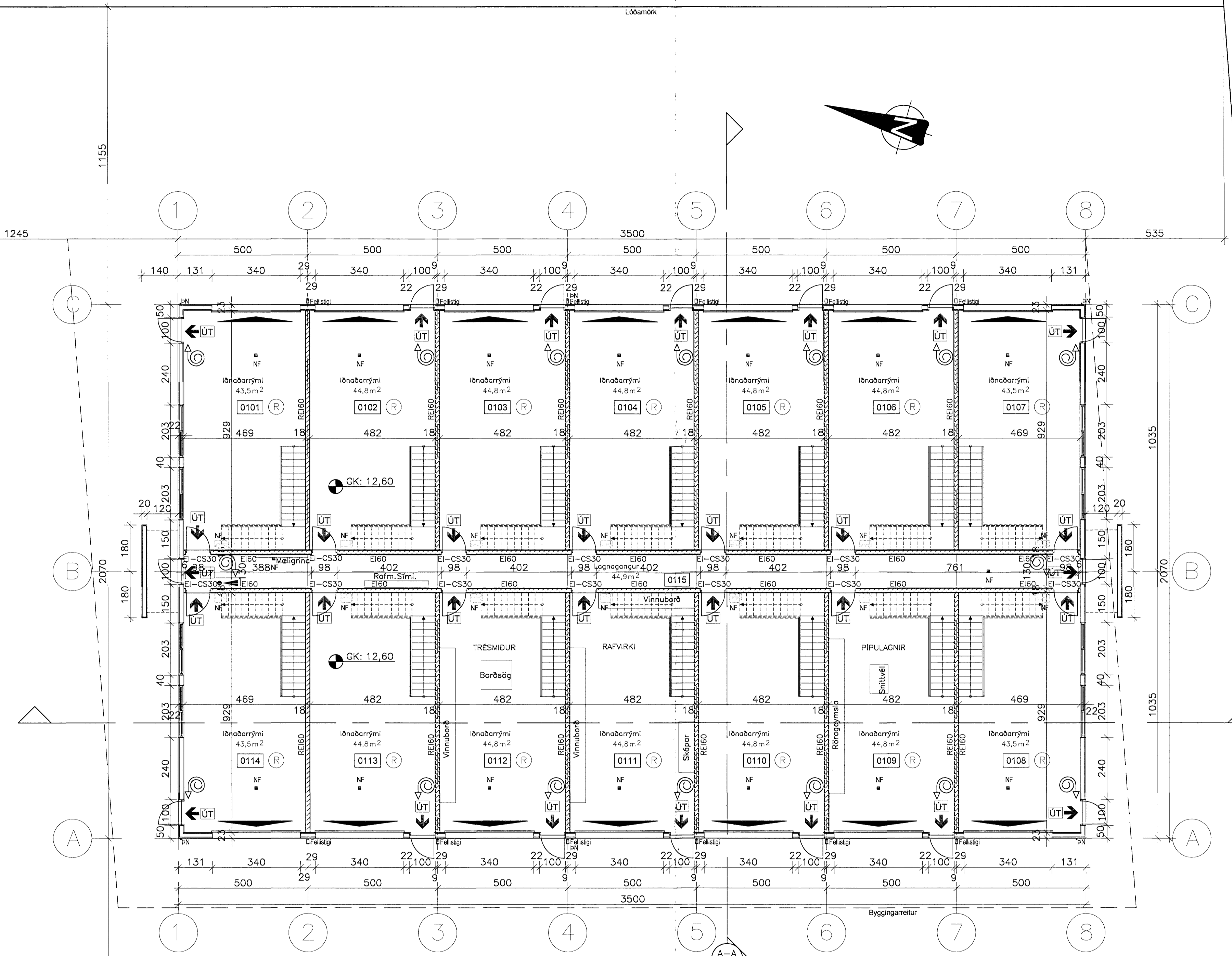
GRUNNMYND 1. HÆÐAR 1:100
