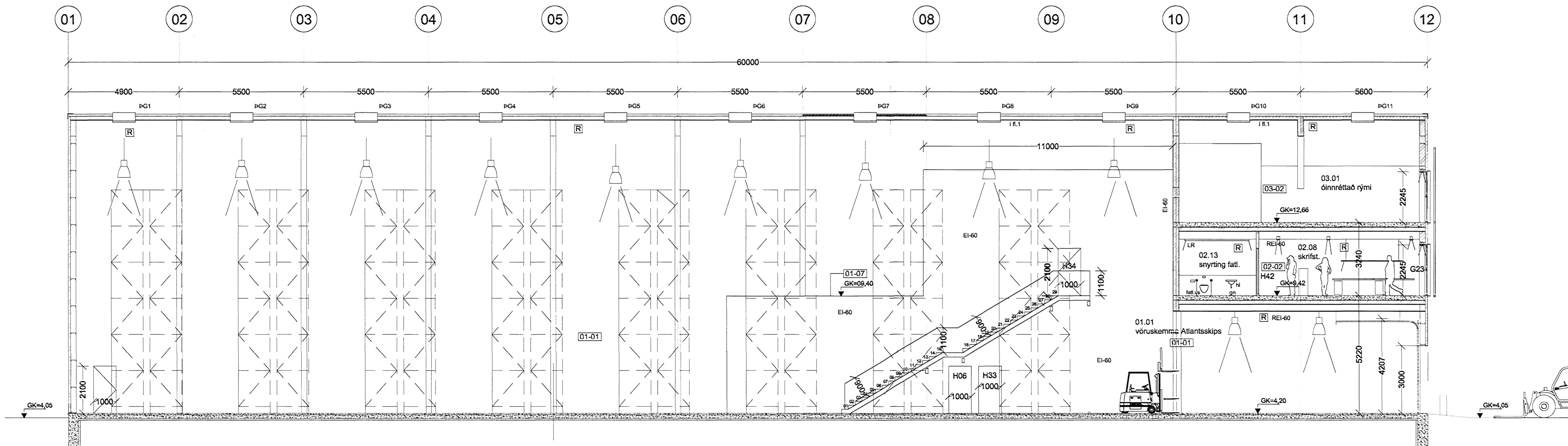
SNEIÐING BB
