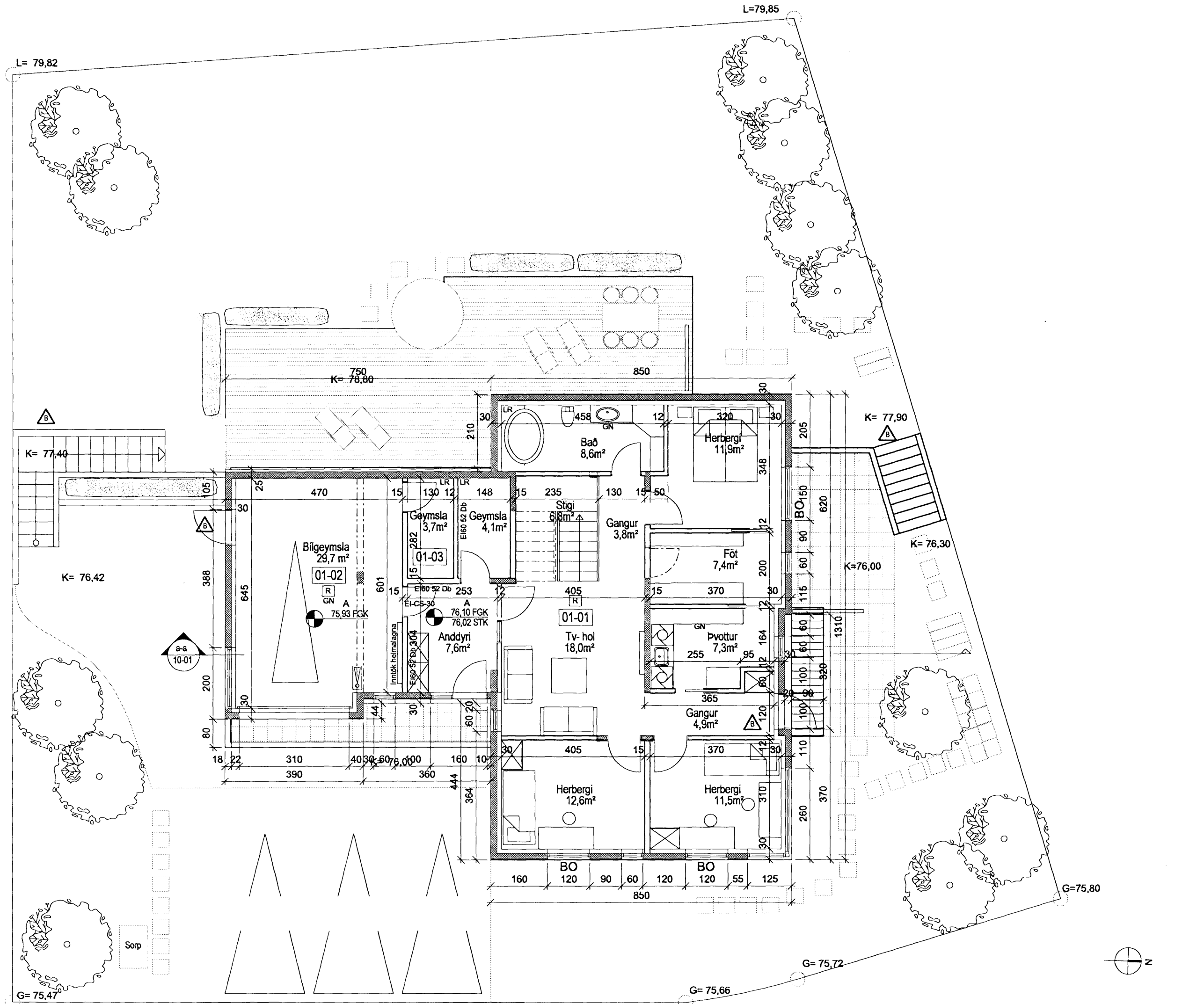
Grunnmynd 1.hæð 1:100
