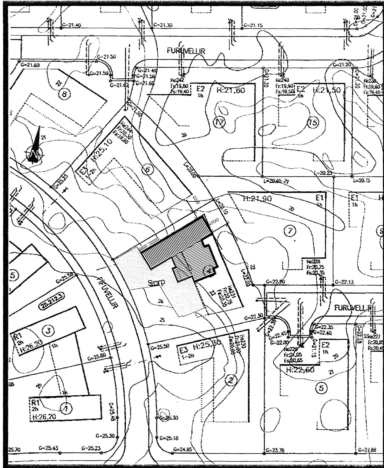
AFSTÖÐUMYND 1:500
