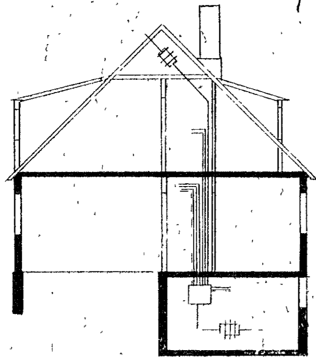
Þverskurður
