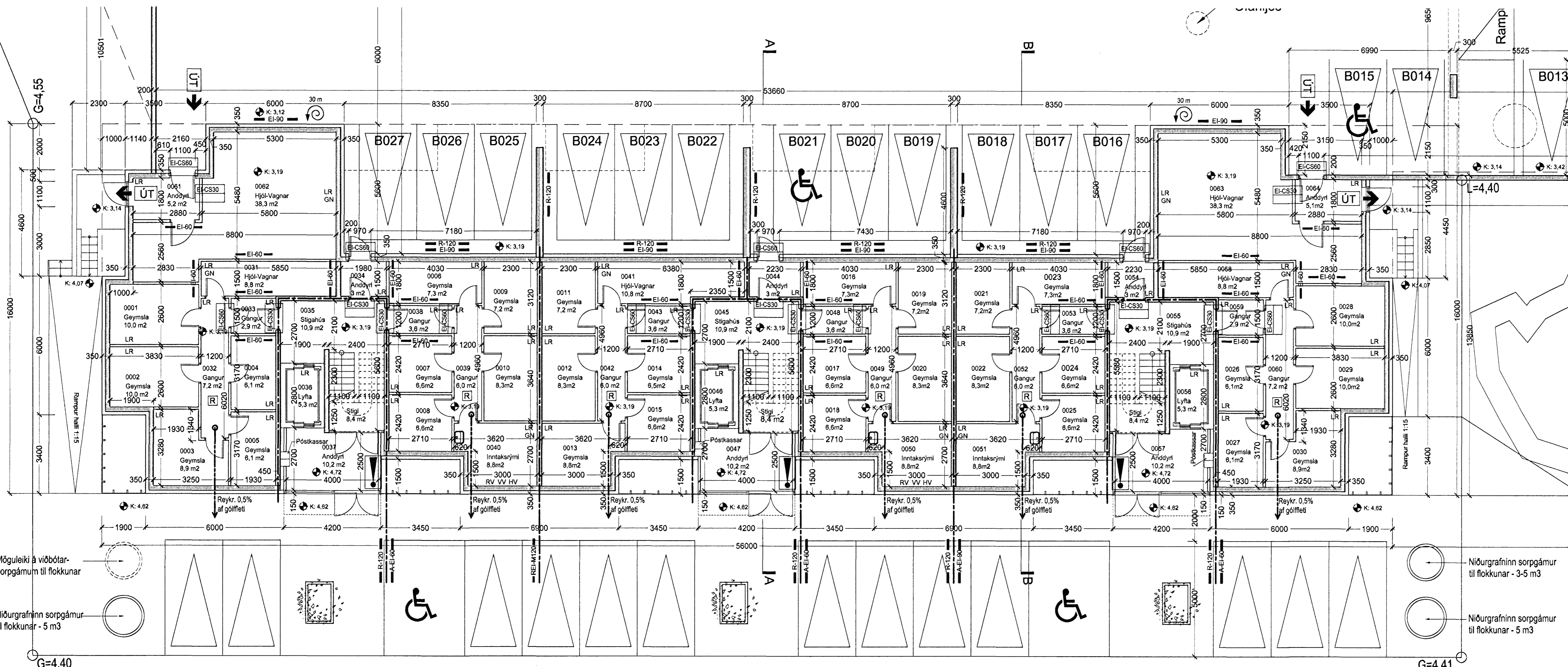
Grunnmynd kjallara í mkv. 1:100
