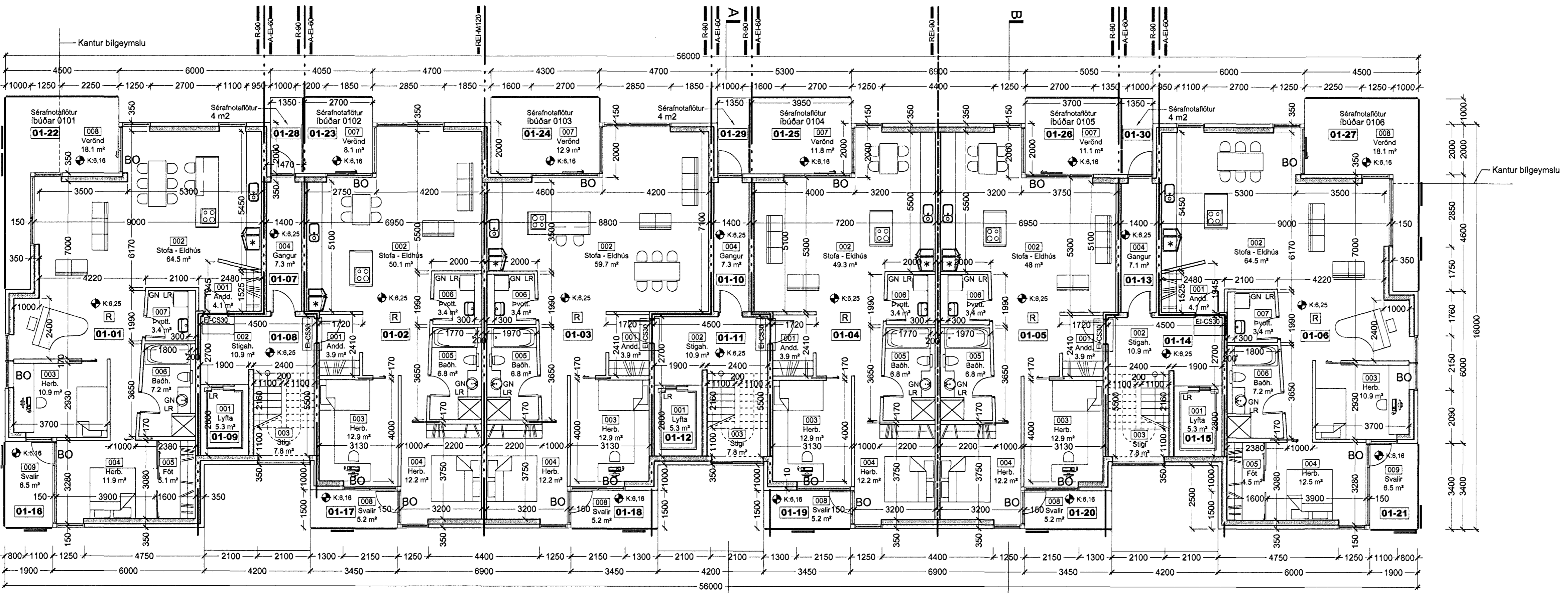
Grunnmynd 1. hæðar í mkv. 1:100
