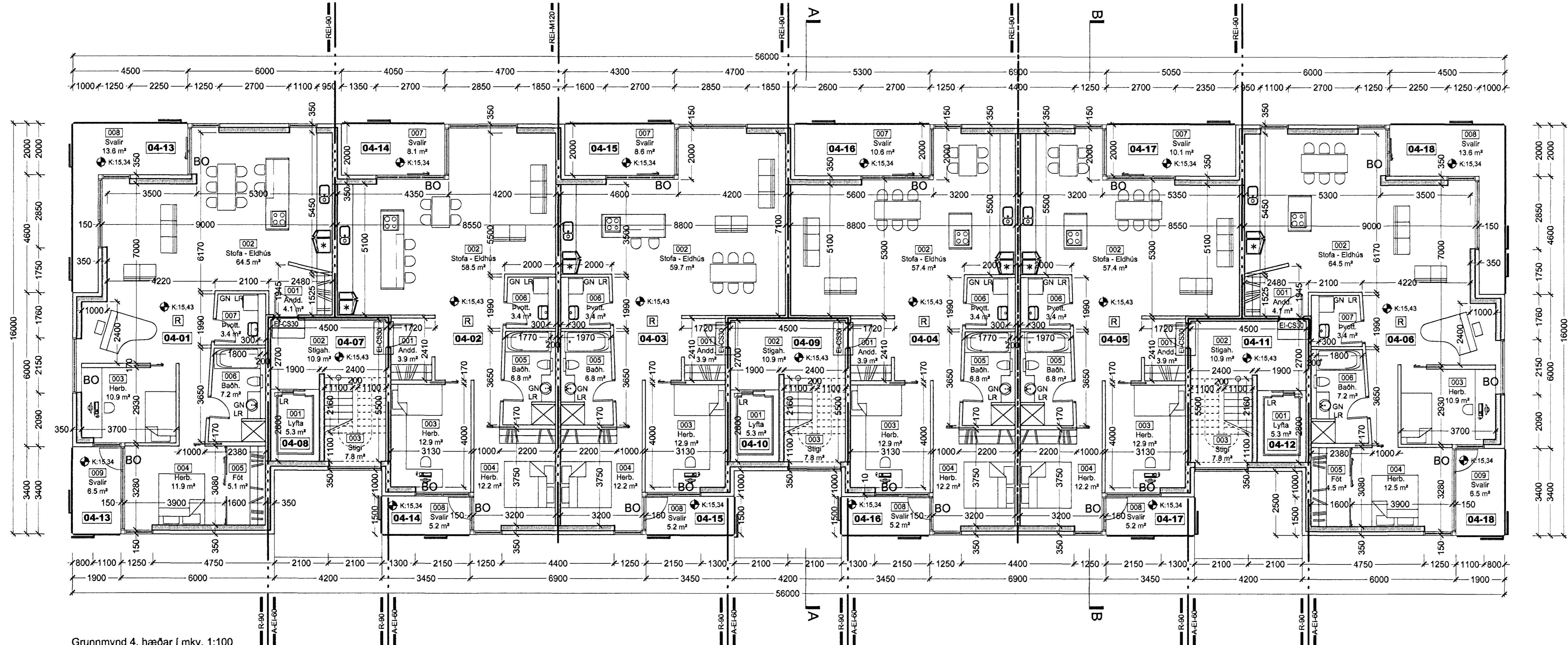
Grunnmynd 4. hæðar í mkv. 1:100
