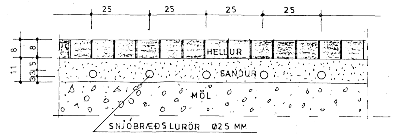
SNIB Í PLAN OG SNJÓBRÆÐSLU M, 1:10
