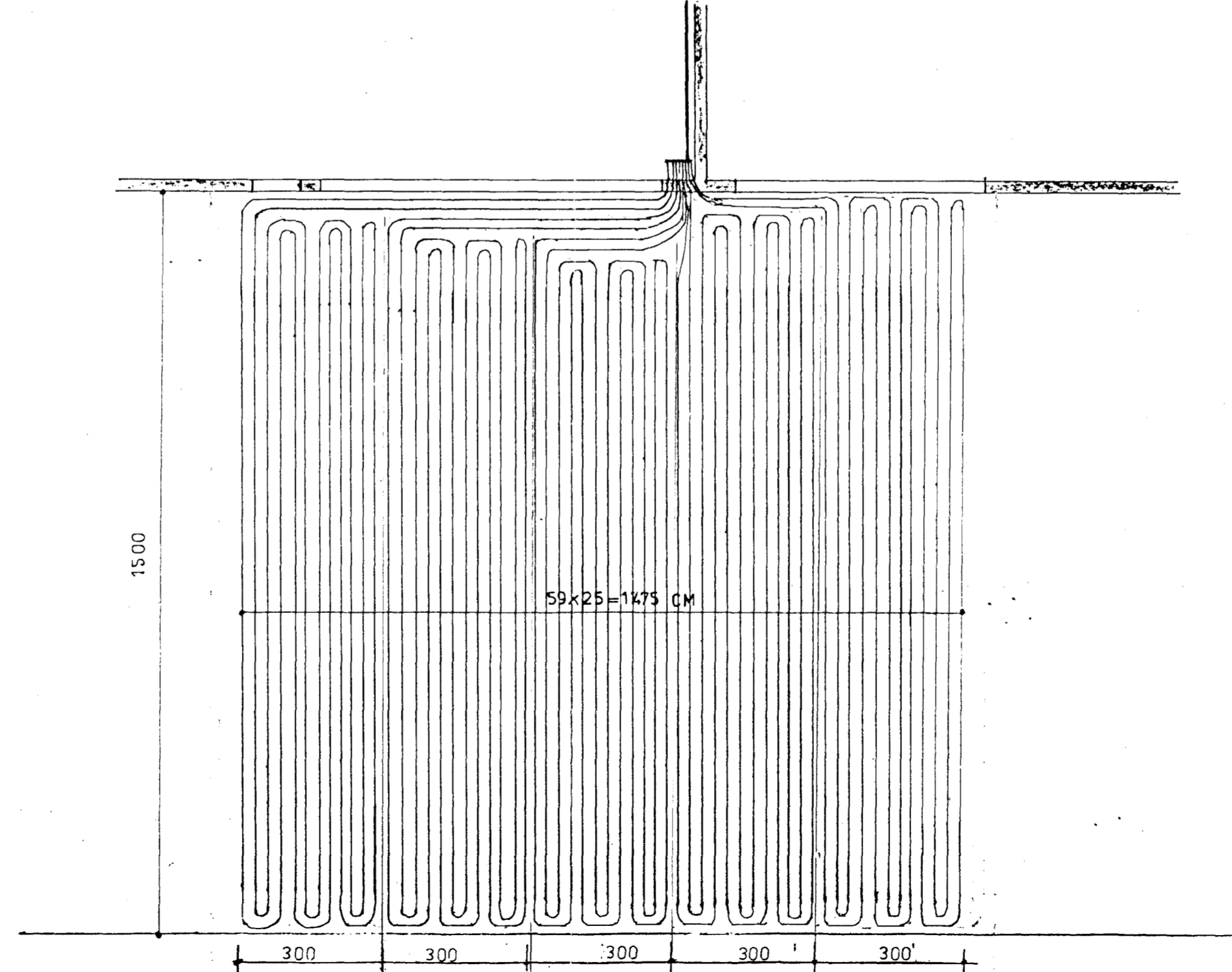
SNIB Í PLAN OG SNJÓBRÆÐSLU M, 1:10
