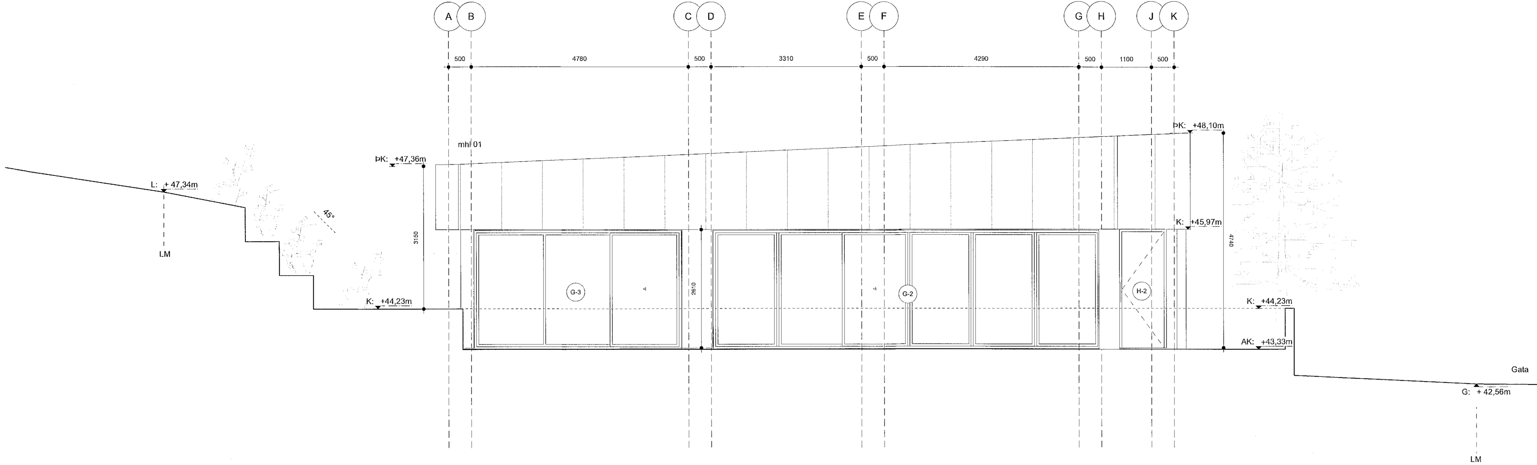
Ásýnd norður mkv: 1:100
