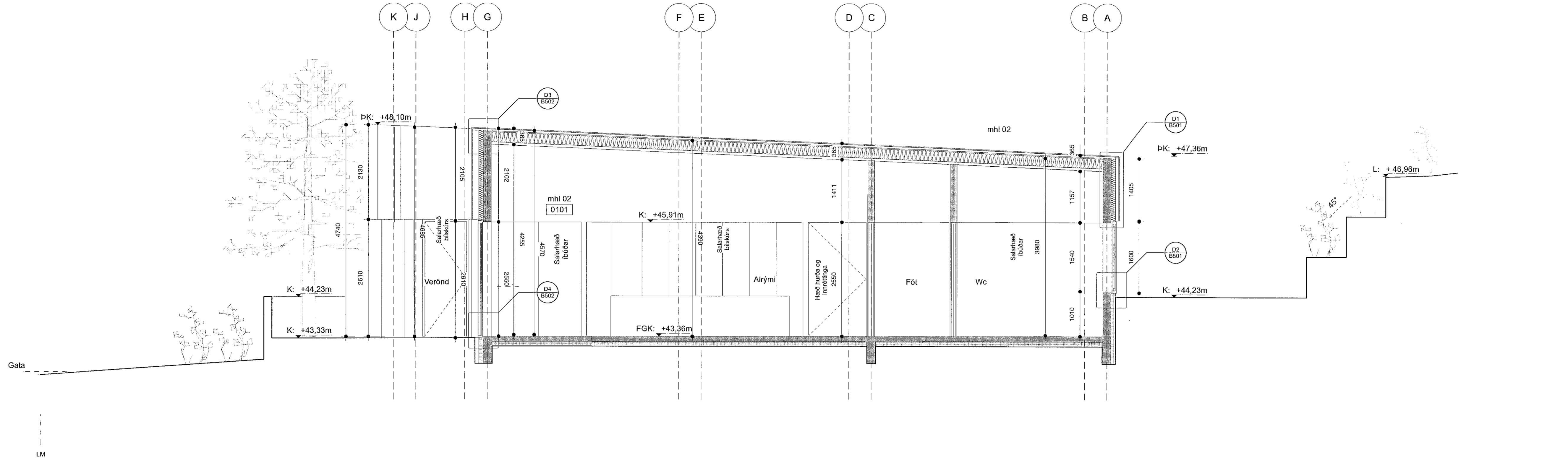
Sneiðing A-A mkv: 1:100
